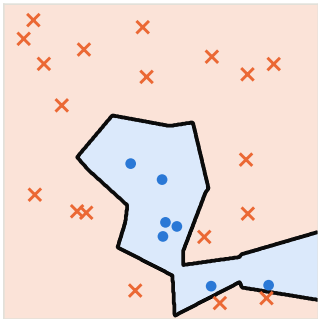
(a) kNN với k=1
