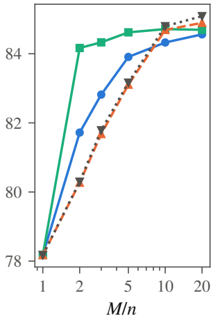
Magic
