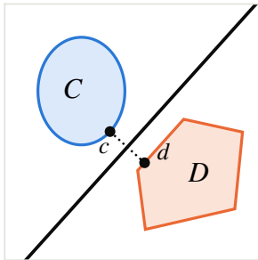
(b) siêu phẳng phân tách
