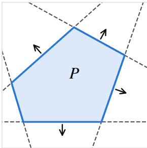
(a) đa diện
