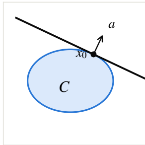
(c) siêu phẳng tựa
