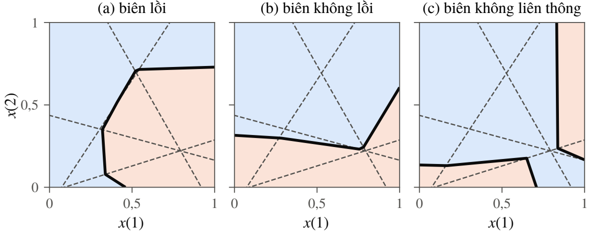
Hình 2.7. Cùng ánh xạ (2.27), ba vectơ trọng số ở Bảng 2.3 cho ba biên (nét liền) có hình dạng rất khác nhau. Nét đứt là bốn đường \varphi_m(x) = 0 , m = 3, \dots, 6 ; vùng tô cam là \{f \leq 0\} . Ví dụ được dựng lại theo ý tưởng của Hình 2 trong [26].
