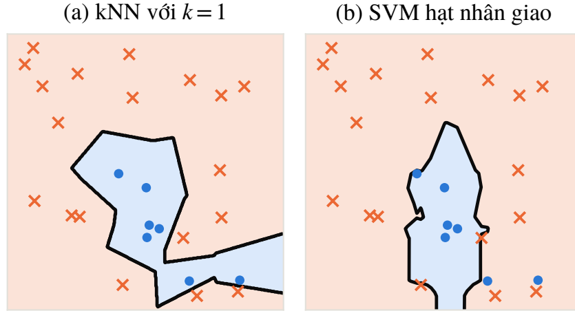
Hình 2.8. Biên quyết định (nét liền) của (a) phương pháp một láng giềng gần nhất và (b) SVM hạt nhân giao trên cùng 26 điểm dữ liệu. Cả hai biên đều tuyến tính từng phần.
