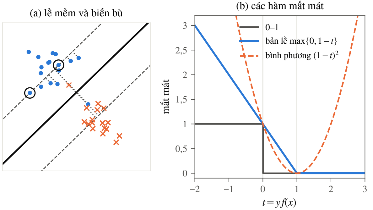
Hình 2.2. (a) SVM lề mềm trên dữ liệu chồng lấn: các điểm vi phạm lề được nối bằng nét chấm tới siêu phẳng lề của lớp mình, độ dài nét chấm bằng e_k/\|w\| ; khoanh tròn là các vectơ hỗ trợ nằm đúng trên lề. (b) Mất mát 0-1, mất mát bản lề của C-SVM và mất mát bình phương của LS-SVM, theo t = yf(x) .
