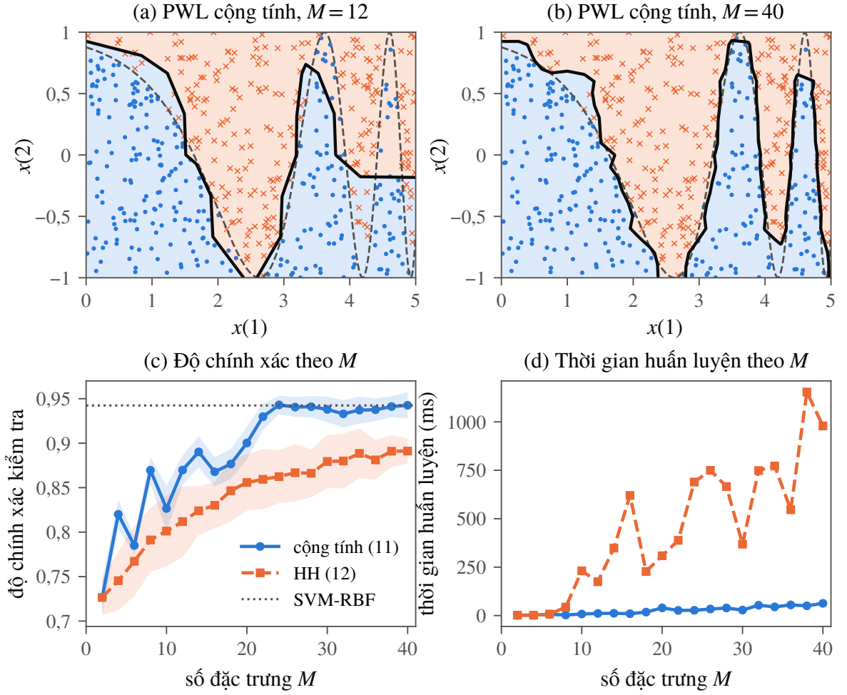
Hình 3.2. Tái hiện thí nghiệm Cosexp (Hình 3 của [26]), 10 lần lặp. (a), (b) Biên của PWL-C-SVM cộng tính với M = 12 và M = 40 (nét liền) so với biên thật (nét đứt). (c) Độ chính xác trên tập kiểm tra theo M : đường là trung bình, dải màu là \pm một độ lệch chuẩn; đường chấm là SVM hạt nhân Gauss. (d) Thời gian huấn luyện (trung vị) với \gamma đã chọn.
