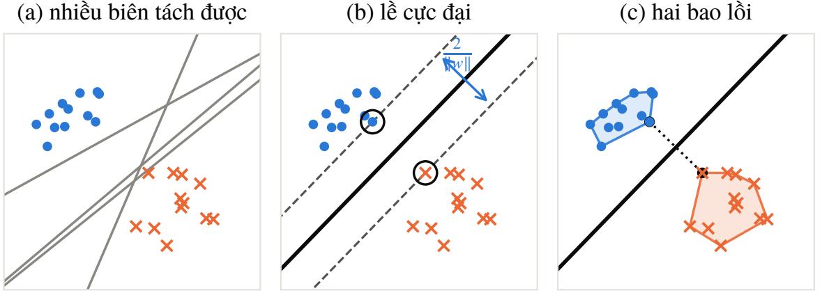
Hình 2.1. SVM lề cứng. (a) Dữ liệu tách được thường có nhiều siêu phẳng phân loại đúng. (b) Siêu phẳng lề cực đại (nét liền), hai siêu phẳng w^\top x + w_0 = \pm 1 (nét đứt) và các vectơ hỗ trợ (khoanh tròn); khoảng cách giữa hai nét đứt là 2/\|w\| . (c) Cách nhìn đối ngẫu: siêu phẳng tối ưu là trung trực của đoạn nối hai điểm gần nhau nhất của hai bao lồi.
