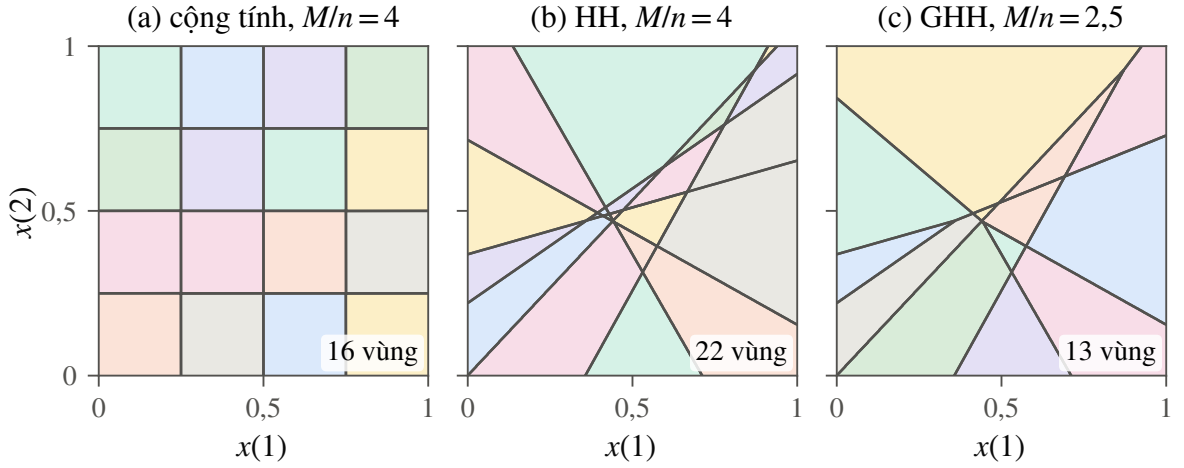
Hình 2.6. Phân vùng tuyến tính của hình vuông đơn vị do ba dạng ánh xạ sinh ra: (a) cộng tính với lưới 4 \times 4 (6 đặc trưng bản lề); (b) HH với 6 siêu phẳng ngẫu nhiên; (c) GHH với 3 đặc trưng, mỗi đặc trưng có 2 siêu phẳng. Trên mỗi vùng, mọi hàm quyết định w^\top \varphi(x) + w_0 đều là hàm affine.
