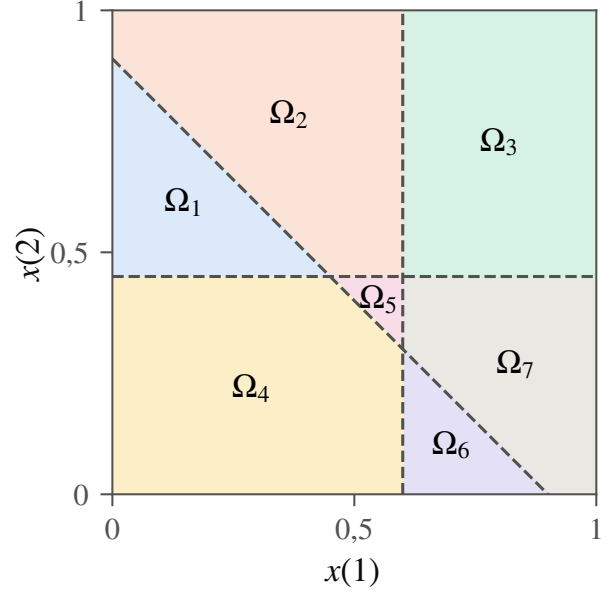
Hình 1.5. Hàm PWL hai biến của Ví dụ 1.24(d). (a) Đồ thị gồm bảy mảnh mặt phẳng nối liền nhau; các nếp gấp nằm trên ba đường thẳng x(1) + x(2) = 0,9 , x(1) = 0,6 và x(2) = 0,45 . (b) Phân hoạch đa diện tương ứng của hình vuông đơn vị.
