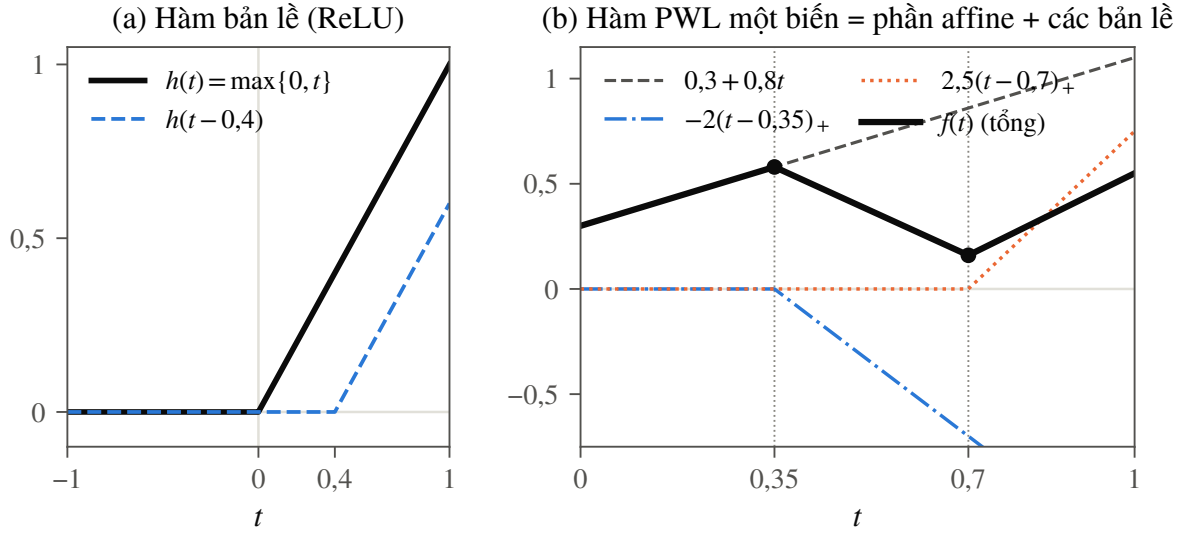
Hình 1.4. (a) Hàm bản lề h(t) = \max\{0, t\} và bản dịch chuyển của nó. (b) Hàm PWL một biến f(t) = 0,3 + 0,8t - 2(t - 0,35)_+ + 2,5(t - 0,7)_+ là tổng của một hàm affine và hai hàm bản lề đặt tại hai điểm gãy; hệ số của mỗi bản lề bằng độ thay đổi hệ số góc tại điểm gãy đó (Mệnh đề 1.27).
