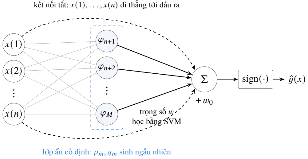
Hình 2.5. PWL-SVM với ánh xạ siêu phẳng bản lề nhìn như một mạng nơ-ron hai lớp: lớp ẩn gồm các nơ-ron ReLU với tham số cố định; các tọa độ x(1), \dots, x(n) đi thẳng đến đầu ra (nét đứt); chỉ các trọng số của lớp ra được học, bằng bài toán lồi (2.16) hoặc (2.20).
