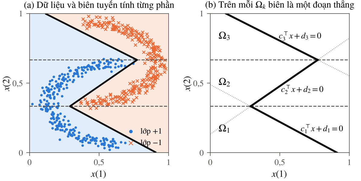
Hình 2.4. Một biên tuyến tính từng phần cho dữ liệu hai mặt trắng ( N = 600 ). (a) Biên gồm ba đoạn thẳng, tách đúng 599/600 điểm. (b) Trên mỗi dải \Omega_k , biên trùng với một đoạn của đường thẳng c_k^T x + d_k = 0 (các phần kéo dài được vẽ bằng nét chấm). Dữ liệu và biên được tính bằng mã của đề án; ý tưởng theo Hình 1 của [26].
