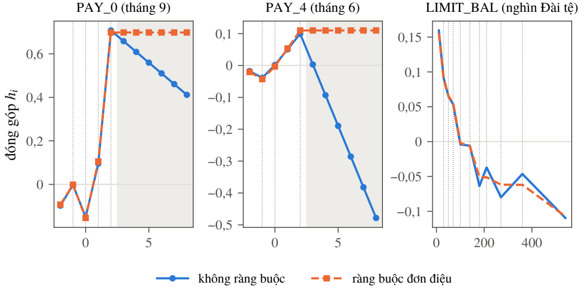
Hình 3.10. Hàm đóng góp của PAY\_0 , PAY\_4 và LIMIT\_BAL trong mô hình không ràng buộc (nét liền) và mô hình có ràng buộc đơn điệu (nét đứt), lần chia đầu tiên. Vùng tô xám: các trạng thái chậm trễ từ ba tháng trở lên, chỉ chiếm chưa tới 2% số khách hàng.
