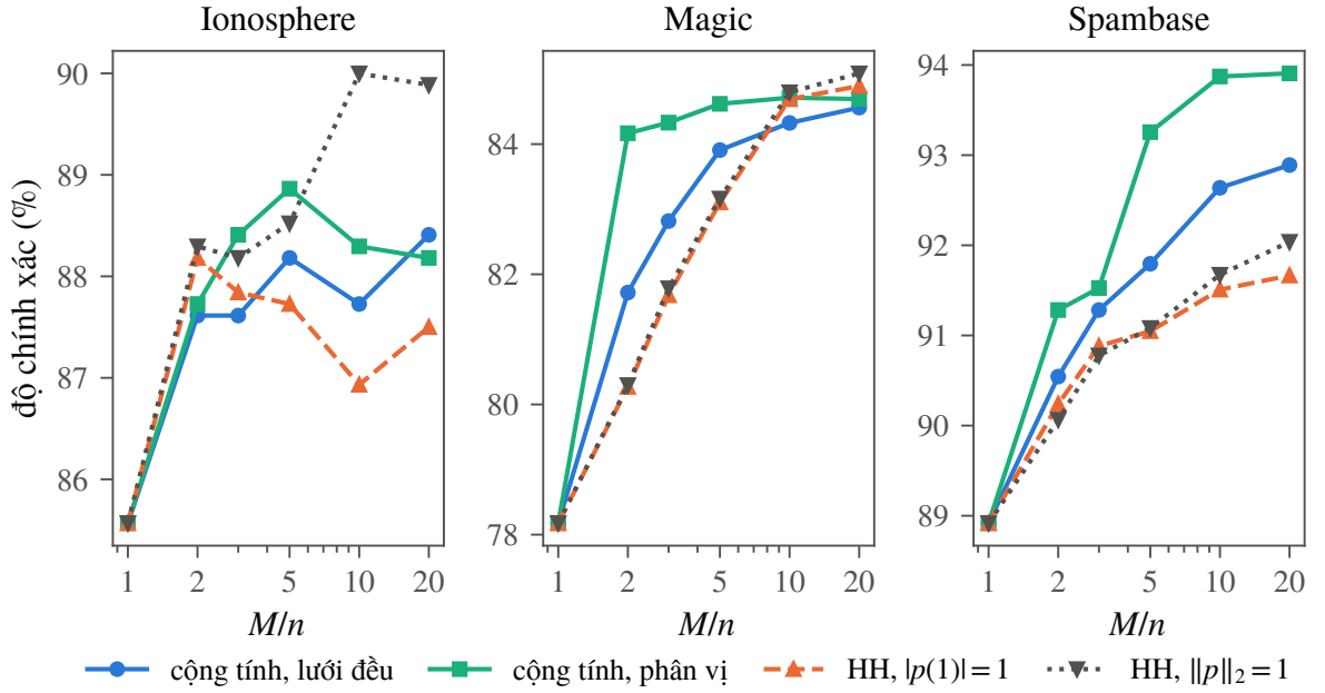
Hình 3.4. Độ chính xác trung bình (qua 5 lần chia) của PWL-LS-SVM theo số đặc trưng trên mỗi chiều M/n , với bốn quy tắc chọn tham số. M/n = 1 ứng với bộ phân loại tuyến tính.
