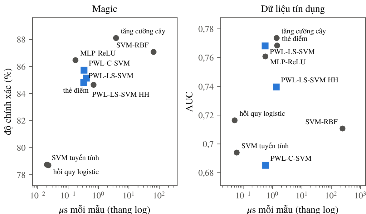
Hình 3.5. Độ chính xác (Magic) hoặc AUC (dữ liệu tín dụng) theo thời gian dự đoán mỗi mẫu, trên thang logarit. Ô vuông là các biến thể PWL-SVM; điểm tròn là các phương pháp khác.
