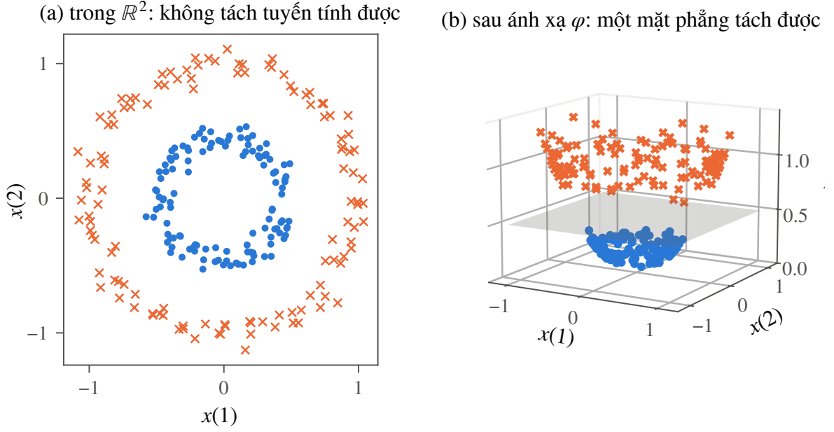
Hình 2.3. (a) Hai vòng tròn đồng tâm không tách tuyến tính được trong \mathbb{R}^2 . (b) Sau ánh xạ \varphi(x) = (x(1), x(2), z) với z = x(1)^2 + x(2)^2 , một mặt phẳng tách được hai lớp.
