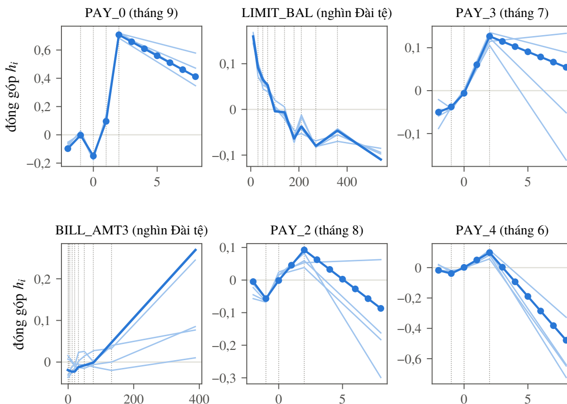
Hình 3.8. Sáu hàm đóng góp h_i có ảnh hưởng lớn nhất của PWL-LS-SVM cộng tính (nút phân vị) trên dữ liệu tín dụng, đã trừ giá trị trung bình. Nét đậm: mô hình của lần chia đầu tiên, nét chấm dọc là vị trí các nút của nó; nét mảnh: mô hình của bốn lần chia còn lại. Giá trị dương ứng với rủi ro vỡ nợ cao hơn.
