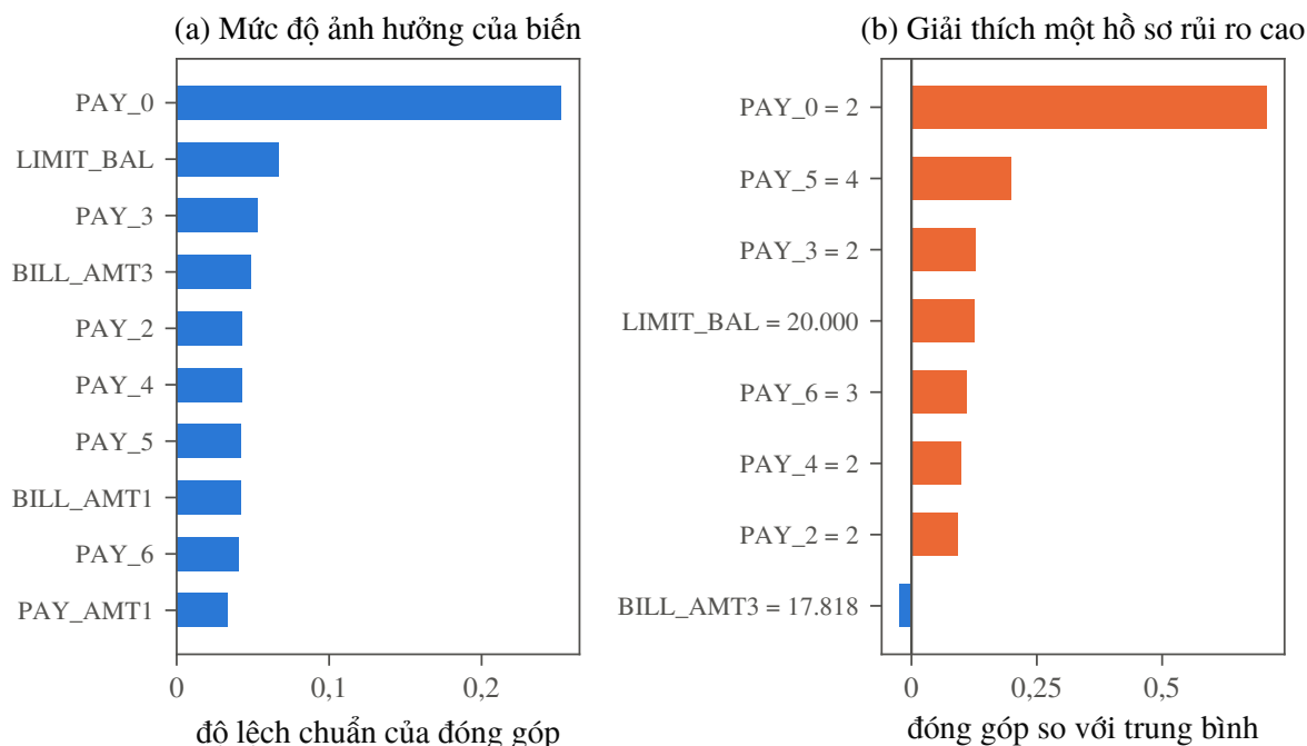
Hình 3.9. (a) Mức độ ảnh hưởng của mười biến quan trọng nhất, đo bằng độ lệch chuẩn của đóng góp h_i trên tập huấn luyện; với các biến định danh, đó là độ lệch chuẩn của tổng đóng góp của các biến chỉ báo tương ứng. (b) Tám đóng góp lớn nhất, so với khách hàng trung bình, của hồ sơ có điểm rủi ro cao nhất trong số các khách hàng vỡ nợ ở tập kiểm tra.
