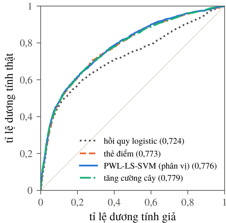
Hình 3.7. Đường cong ROC trên tập kiểm tra của lần chia đầu tiên cho bốn mô hình; con số trong ngoặc là AUC trung bình qua năm lần chia.
