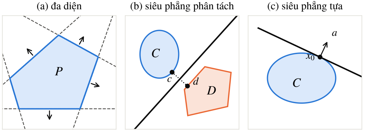
Hình 1.2. (a) Đa diện P là giao của năm nửa không gian; mũi tên chỉ vectơ pháp tuyến a_j hướng ra ngoài. (b) Siêu phẳng phân tách hai tập lồi rời nhau C và D , dựng từ cặp điểm gần nhau nhất c \in C, d \in D như trong chứng minh Định lý 1.8. (c) Siêu phẳng tựa của tập lồi C tại điểm biên x_0 .
