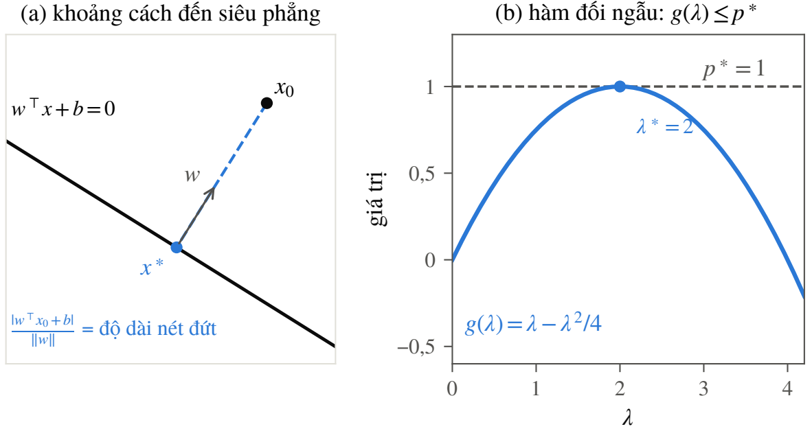
Hình 1.3. (a) Hình chiếu x^* của điểm x_0 lên siêu phẳng w^\top x + b = 0 (Ví dụ 1.19). (b) Hàm đối ngẫu của Ví dụ 1.20 luôn nằm dưới giá trị tối ưu p^* và chạm tới p^* tại \lambda^* = 2 .
