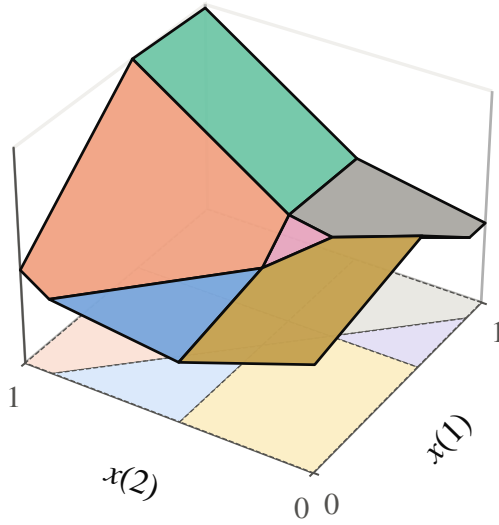
(a) Đồ thị của f : các mảnh phẳng nối liền
