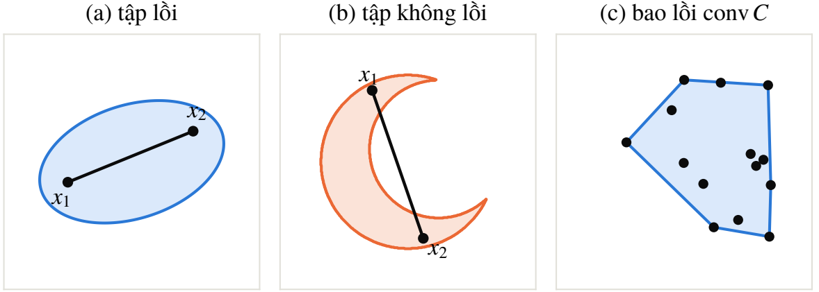
Hình 1.1. (a) Một tập lồi: đoạn thẳng nối hai điểm bất kỳ nằm trọn trong tập. (b) Một tập không lồi. (c) Bao lồi của một tập hữu hạn điểm là đa giác lồi nhỏ nhất chứa các điểm đó.
