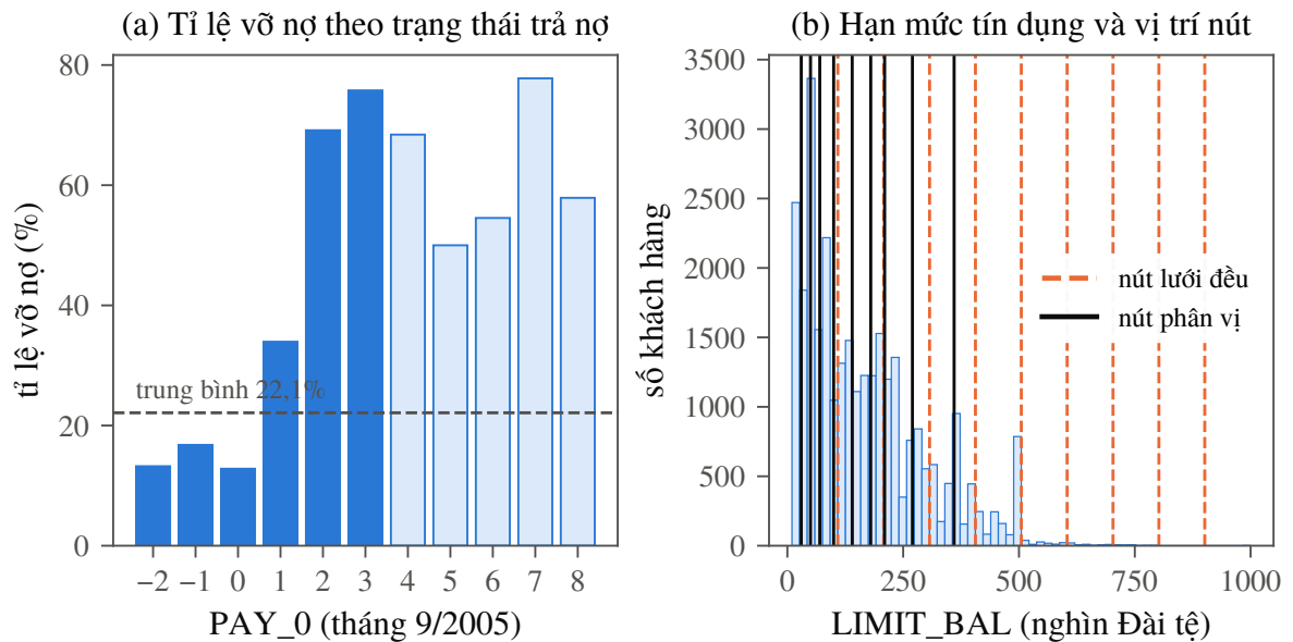
Hình 3.6. (a) Tỷ lệ vỡ nợ theo trạng thái trả nợ tháng 9 (PAY_0); cột nhạt ứng với các nhóm có ít hơn 100 khách hàng. (b) Phân bố hạn mức tín dụng cùng vị trí 9 nút của lưới đều (nét đứt) và của lưới theo phân vị (nét liền).
