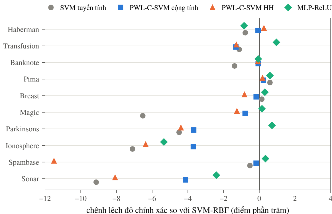
Hình 3.3. Chênh lệch độ chính xác trung bình so với SVM hạt nhân Gauss (điểm phần trăm; giá trị âm nghĩa là kém hơn) của bốn phương pháp trên mười bộ dữ liệu.
