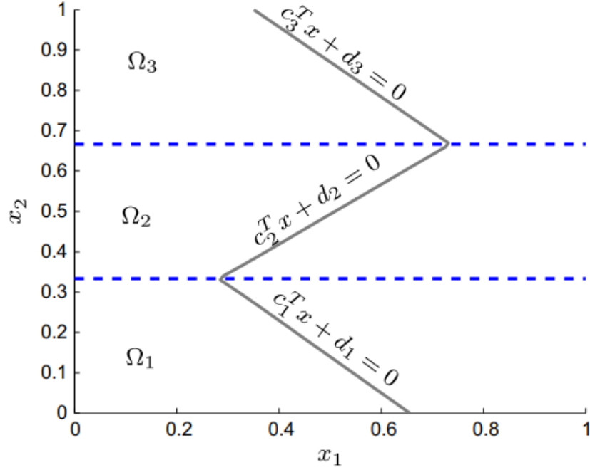
Hình 4: Biên phân loại bị giới hạn trong mỗi vùng con, ranh giới tuyến tính từng phần tương ứng với một đường thẳng.
