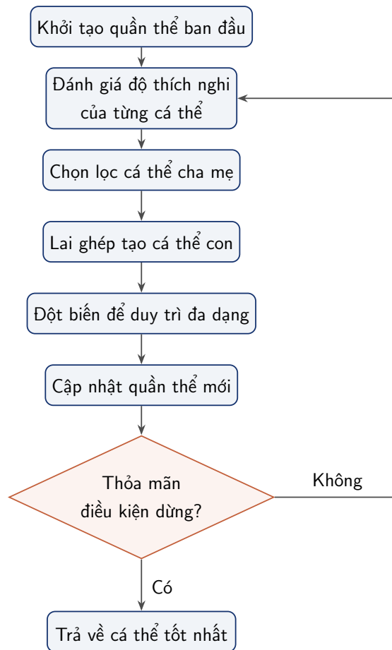
Hình 2.3.1: Sơ đồ tổng quát của Giải thuật Di truyền
