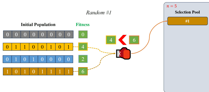
Hình 2.6.1: Minh họa quá trình chọn lọc dựa trên giá trị fitness
