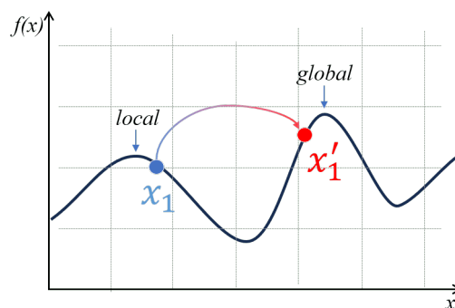
Hình 2.7.1: Minh họa vai trò của đột biến trong duy trì đa dạng di truyền
