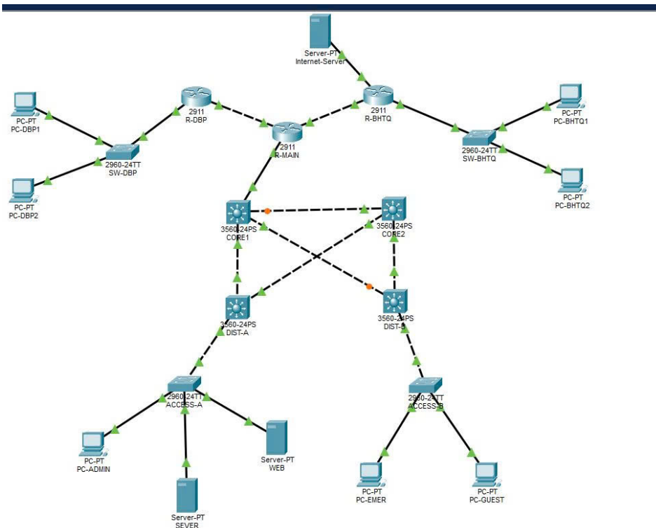
Hình 4.1: Sơ đồ thực thể mạng mô phỏng trên Cisco Packet Tracer
