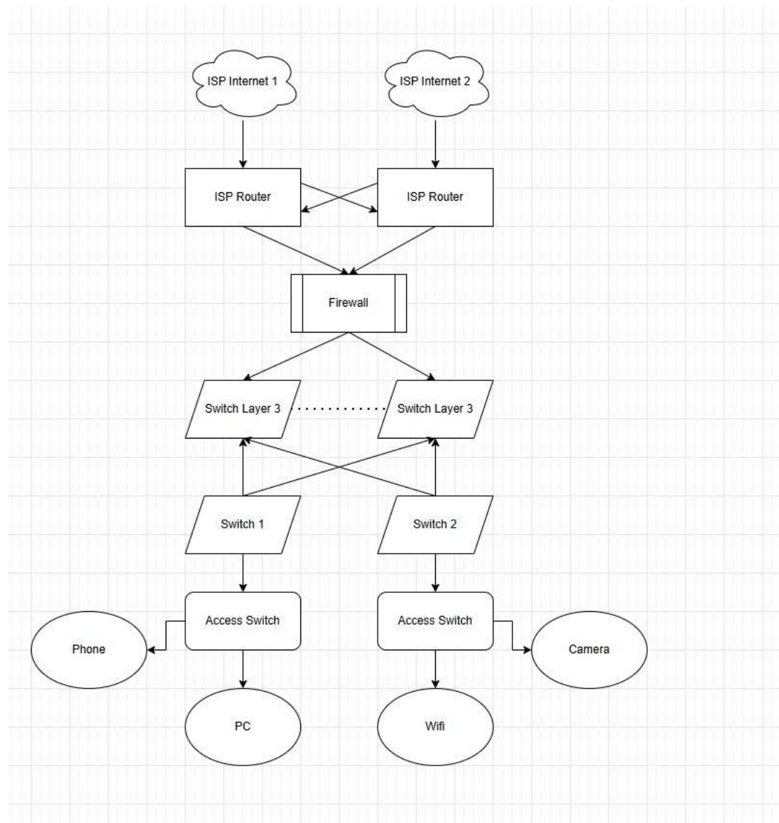
Hình 1.1: Sơ đồ mô hình mạng phù hợp cho bệnh viện
