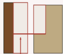
CT 2 — khe luồn ngón. TL 5,6:1
