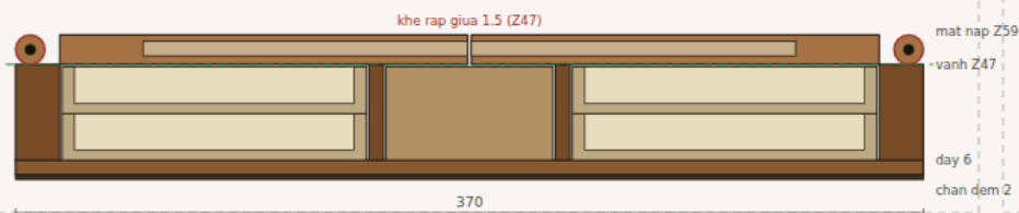
MAT CAT B-B — cat dọc tại X = 165, qua giữa hốc am. TL 1,62:1
