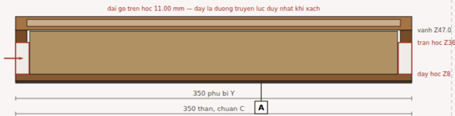
MAT CAT B-B — cat dọc tại X = 165, qua giữa hốc am. TL 1,62:1
