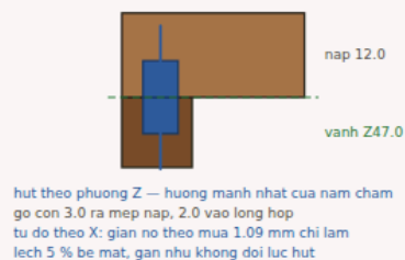
C · Mặt cắt qua một cặp nam châm TL 4.6:1
