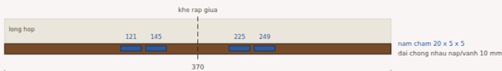
B · Bố trí nam châm — nhìn từ trên, dài mép trước. TL 1,5:1
