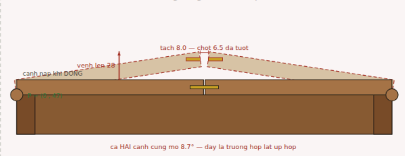
A · Vì sao khóa nối CÁNҺ với CÁNҺ không dùng được — TL 1,5:1
