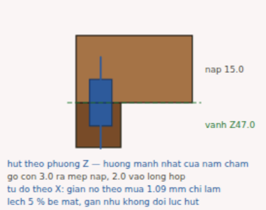
C · Mặt cắt qua một cặp nam châm TL 4.6:1
