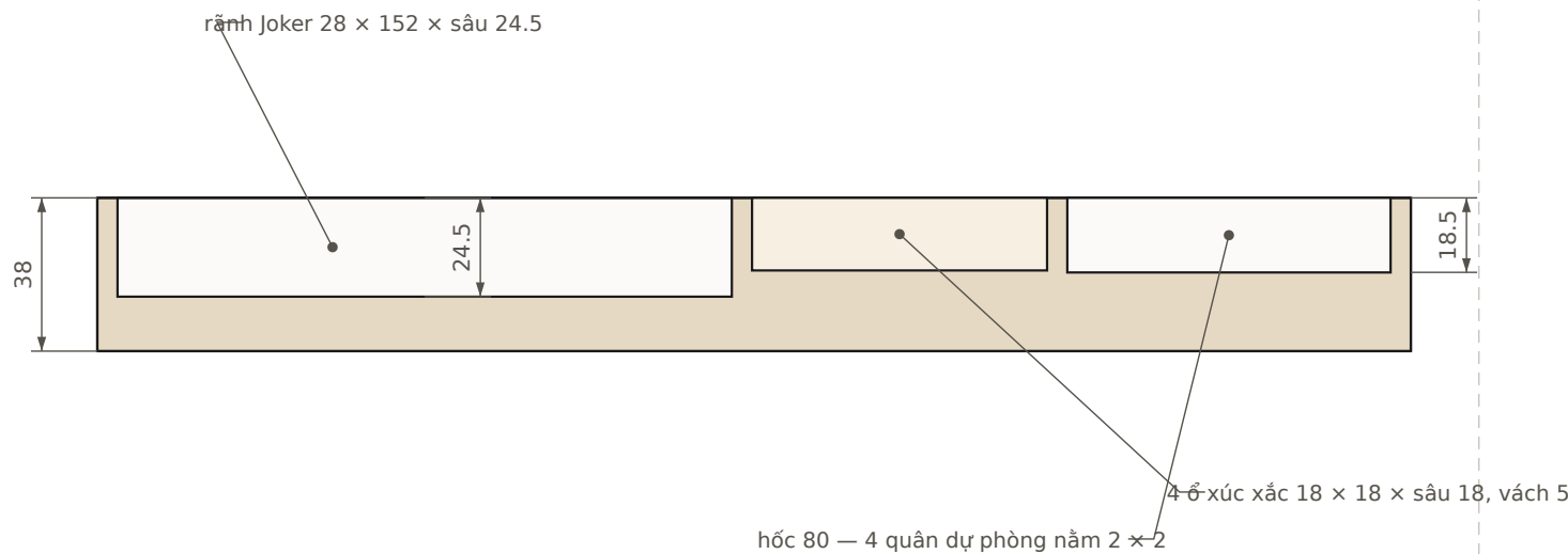
MẶT CẮT DỌC AC-01
