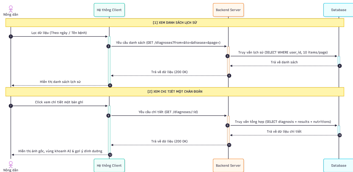
Hình 9: Biểu đồ tuần tự: Tra cứu lịch sử và xem chi tiết
