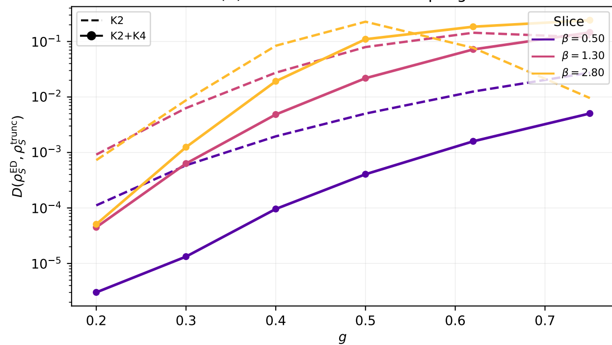
(D) Rescaled cumulants (coupling collapse)
