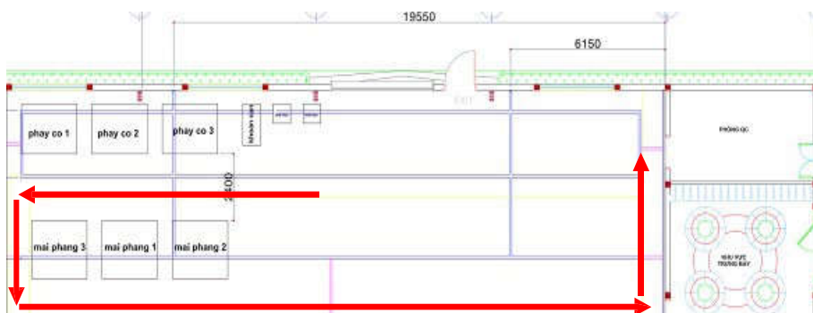
Hình 6.6: Đường di chuyển của Mizusumashi cho công đoạn Tạo phôi
