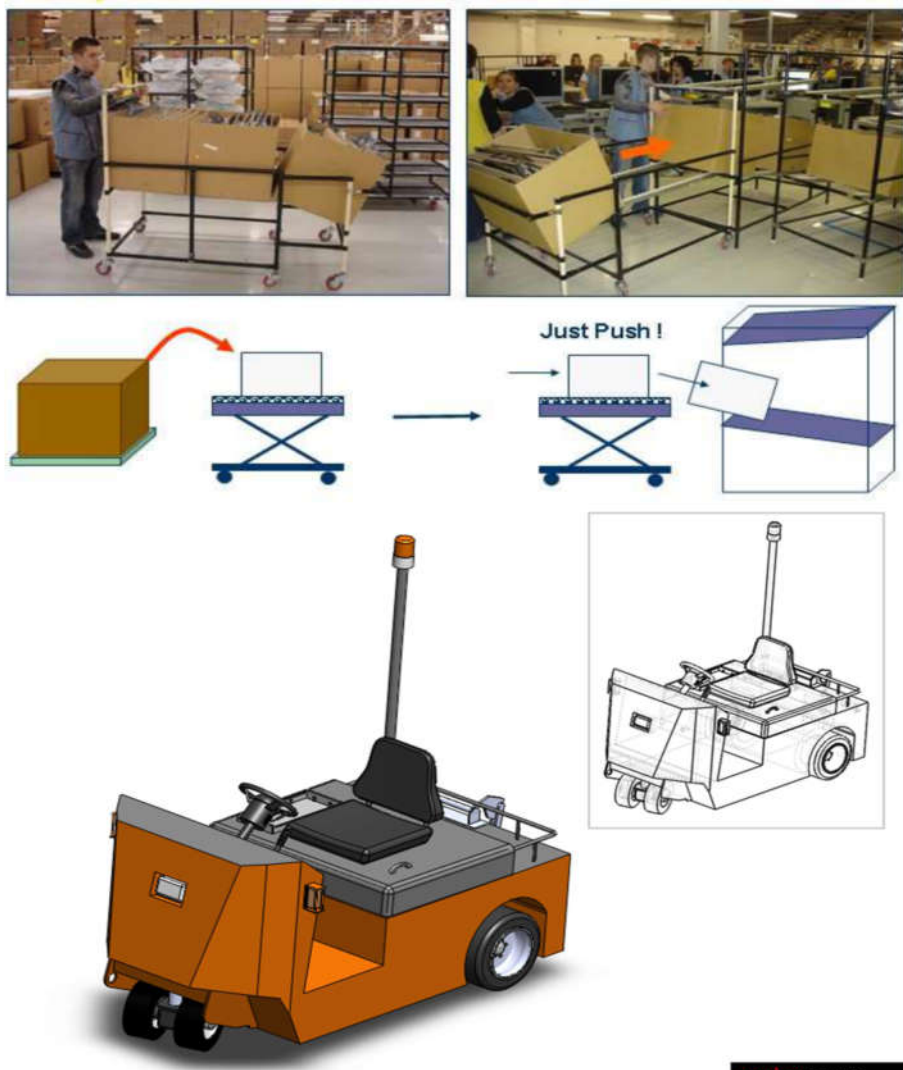
Hình 4.9a: Các dụng cụ, thiết bị hỗ trợ cho Mizusumashi
