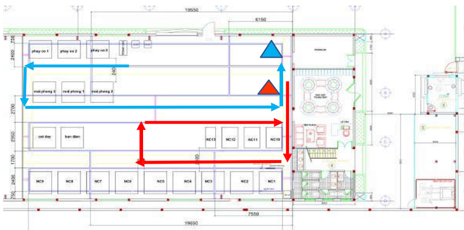
Hình 6.8: Đường di chuyển cuối cùng của 2 Mizusumashi
