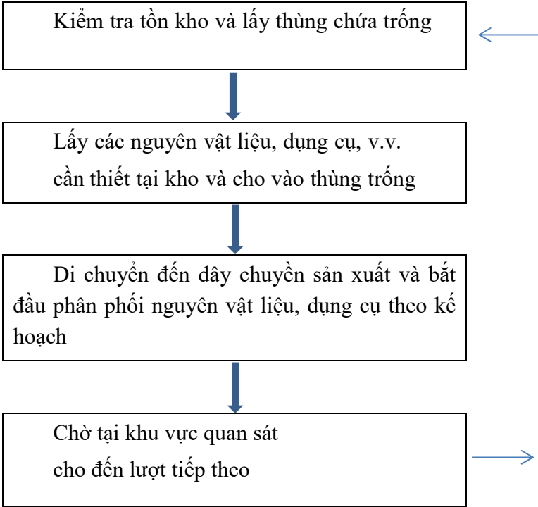
Hình 4.4: Quy trình làm việc của Mizusumashi
