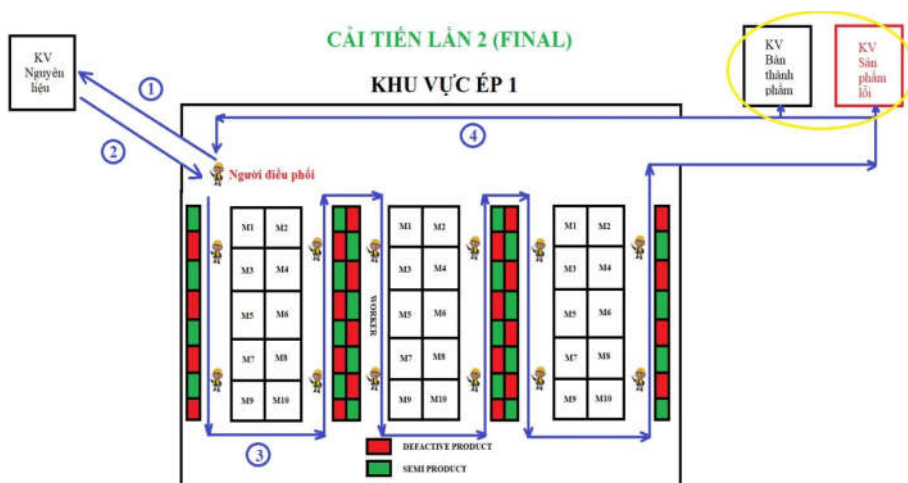
Hình 6.15: Sơ đồ thiết kế (lần 2) đường di chuyển của Mizusumashi
