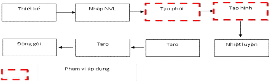
Hình 6.4: Sơ đồ quá trình gia công sản phẩm cơ khí chính xác
