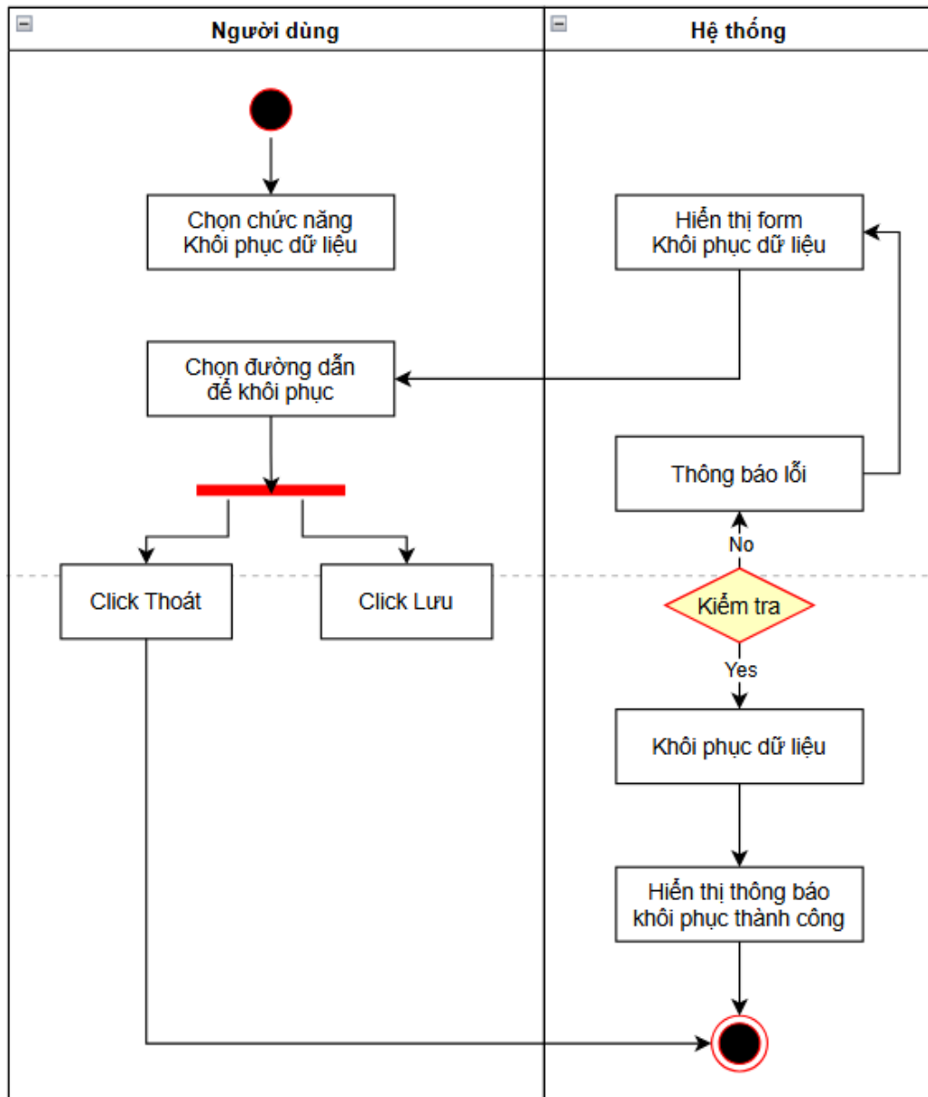
Hình 3.18: Biểu đồ hoạt động “Khôi phục dữ liệu”
