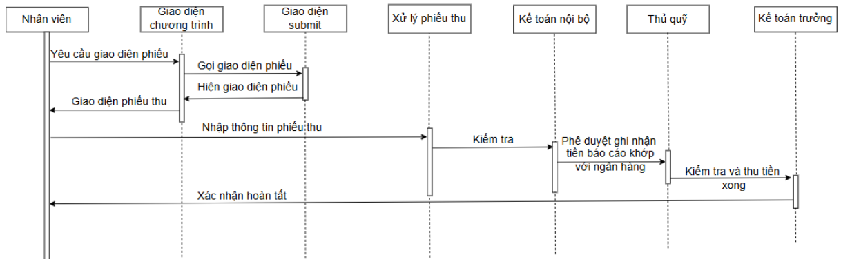
Hình 3.14: Biểu đồ tuần tự quản lý phiếu thu
