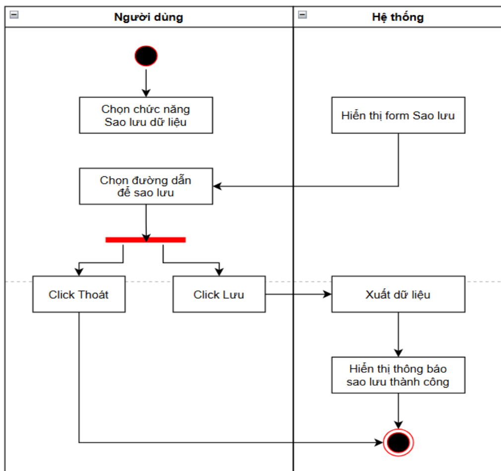
Hình 3.17: Biểu đồ hoạt động “Sao lưu dữ liệu”
