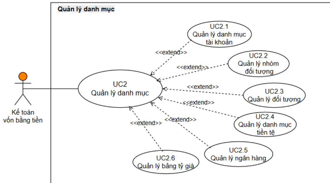
Hình 3.4: Use Case Quản lý danh mục
