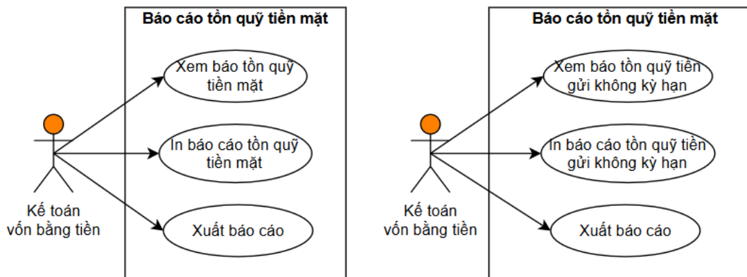
Hình 3.8: Use Case Quản lý Báo cáo
