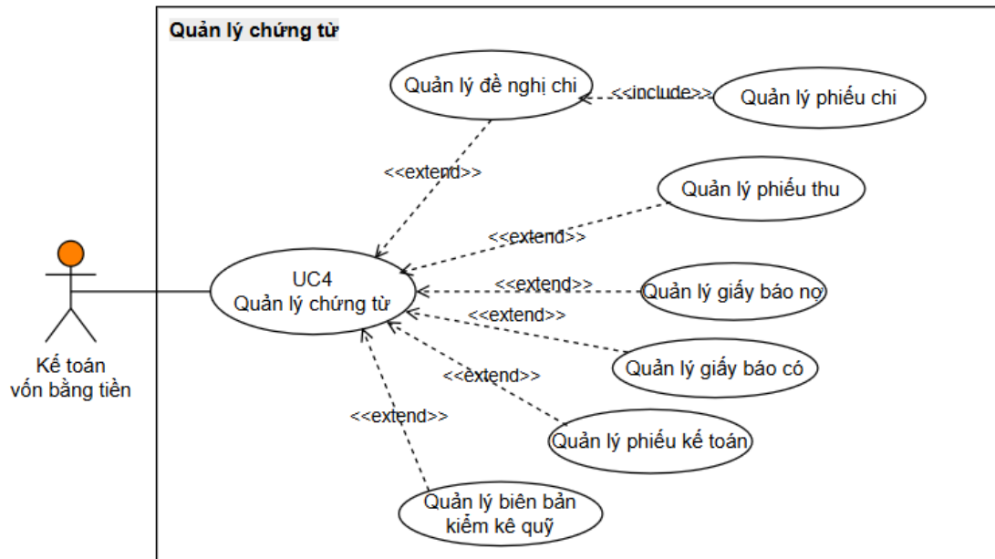
Hình 3.6: Use Case Quản lý chứng từ
