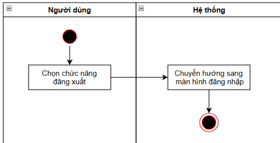
Hình 3.16: Biểu đồ hoạt động “Đăng xuất”
