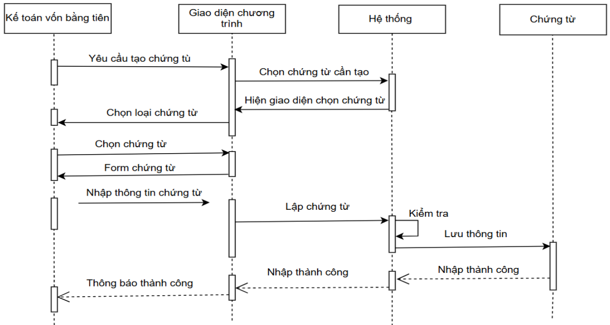
Hình 3.11: Biểu đồ tuần tự “Tạo/ Cập nhật thông tin chứng từ”
