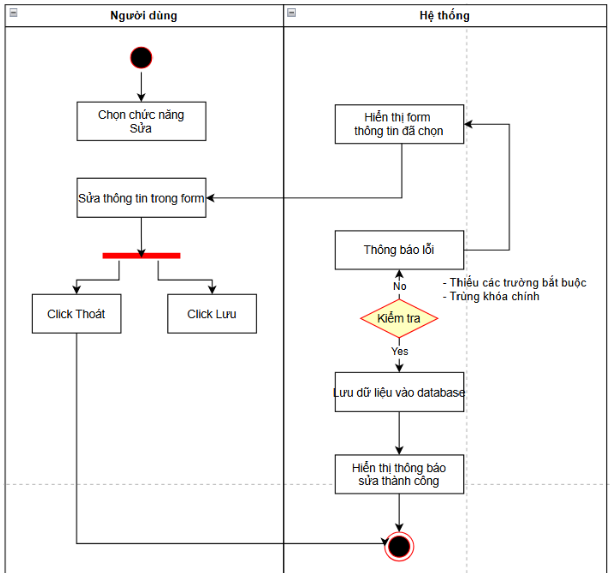
Hình 3.20: Biểu đồ hoạt động “Sửa thông tin”
