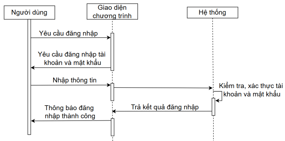
Hình 3.10: Biểu đồ tuần tự “Đăng nhập”
