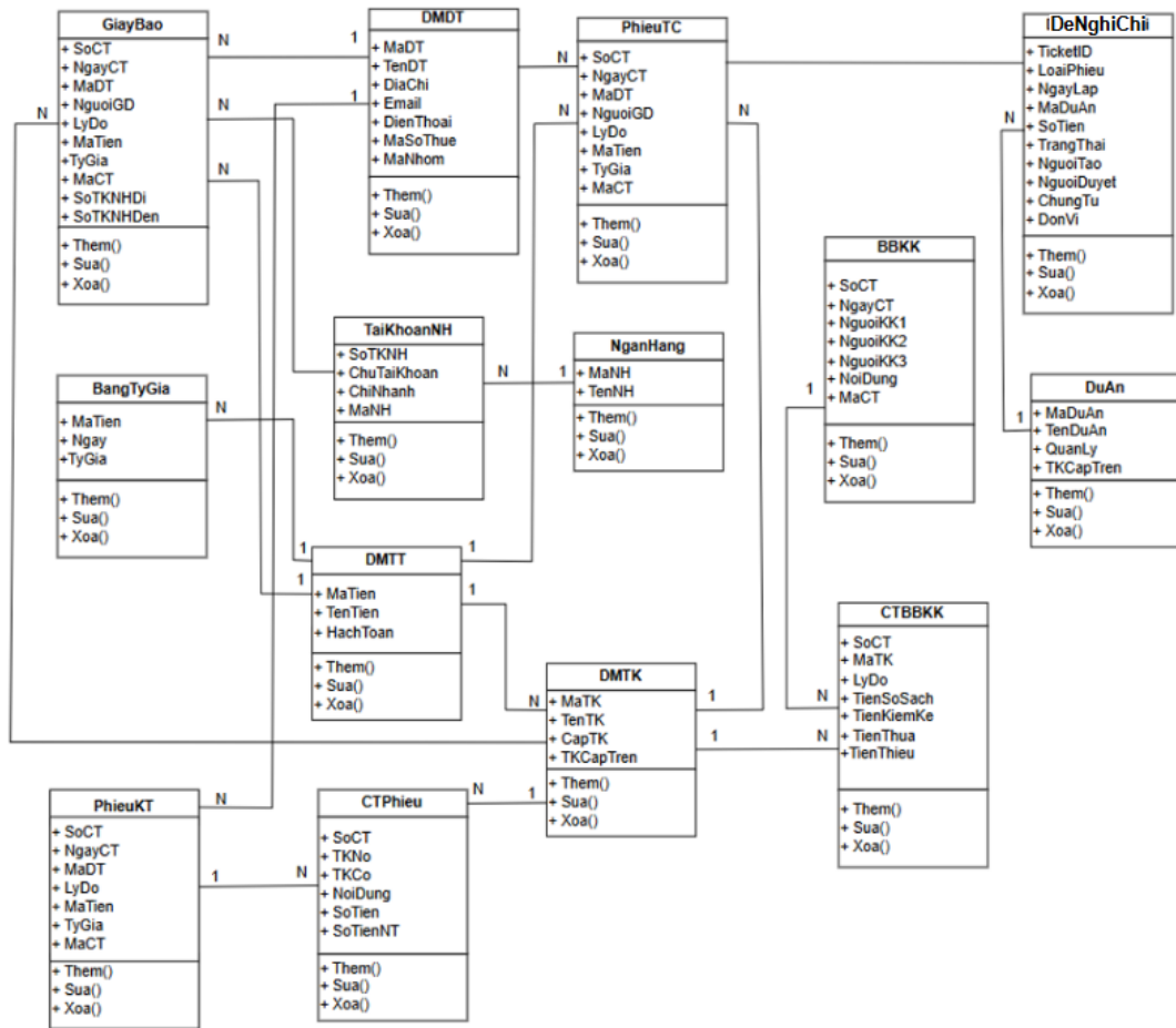
Hình 3.9: Biểu đồ lớp (Class Diagram)
