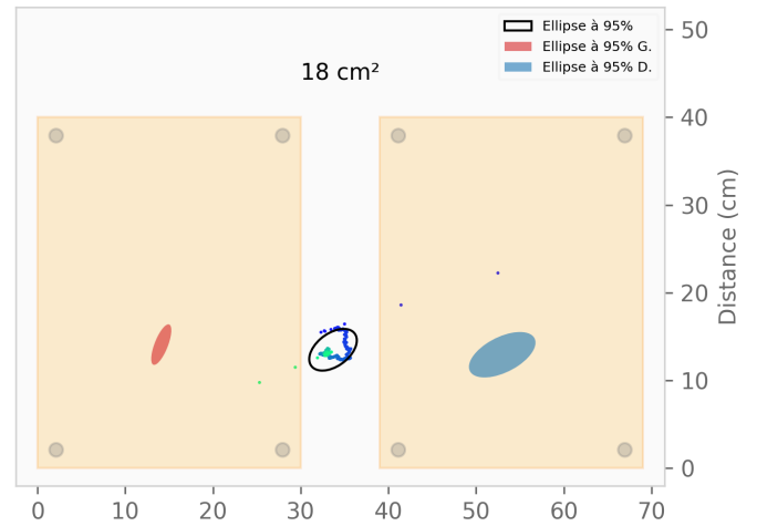
Essai 3 : Déplacement du CoP
