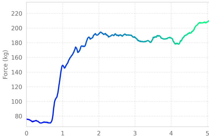
Essai 2 : Force totale
