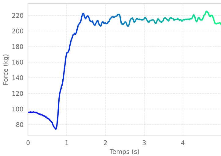
Essai 3 : Force totale
