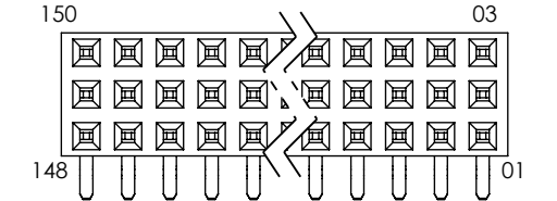
-S, -P, -S-RA & -P-RA
