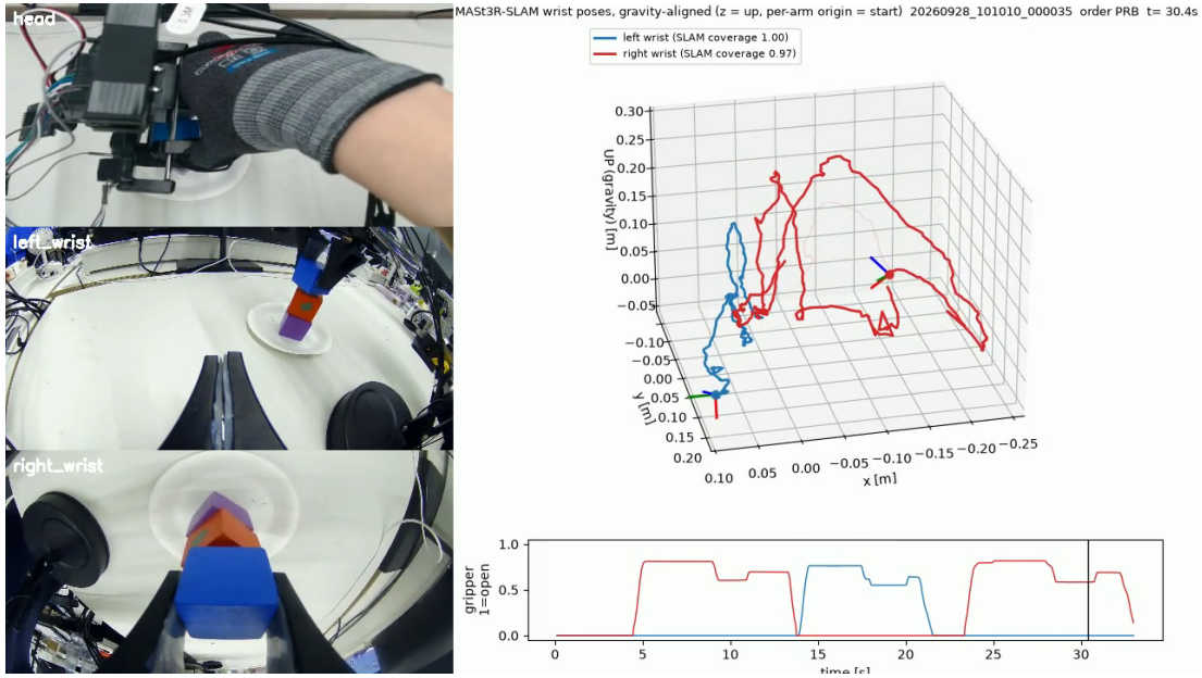
Fig. 4. HRL80 썬치 테이크(순서 PRB)의 MAST3R-SLAM 손목 궤적. 왼쪽: 헤드 카메라와 두 손목 어안 카메라. 오른쪽: 중력 정렬( z 위쪽)된 궤적으로, 각 팔의 원점은 시작 자세이고 현재 공구 축을 표시( x 빨강, y 초록, z 파랑)하며 매트릭 스케일은 IMU에서 얻었다. 아래: 두 그리퍼( 1 = 열림). 세 테이크(PRB, RBP, PBR)의 영상은 저장소의 docs/media/mast3r_trajectories/hr180_0000{35,55,60}_wrist.mp4에 있다.
