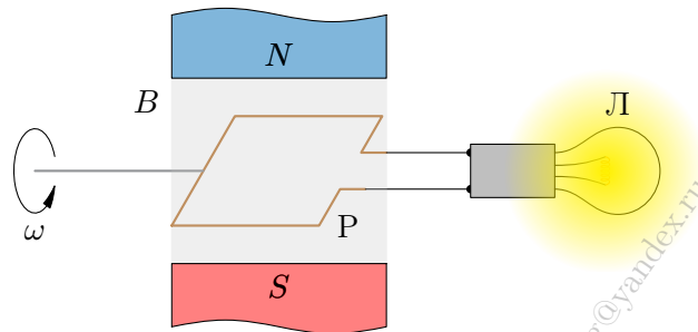
Рис. 166. Схема генератора переменного тока
