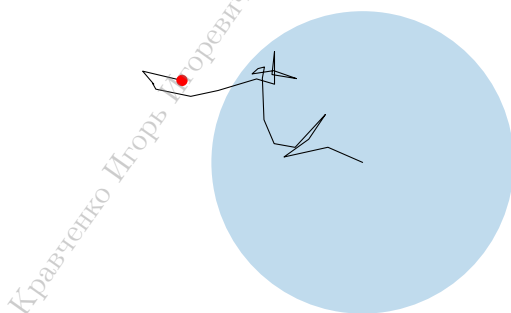
Рис. 65. Броуновское движение
