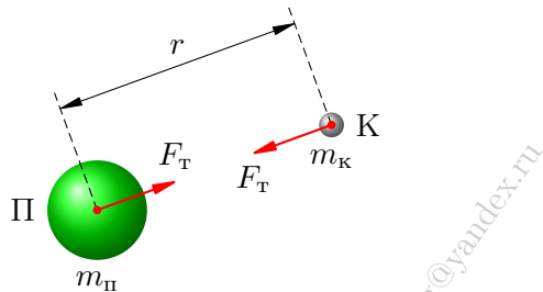
Рис. 34. Притяжение планеты и космического корабля
