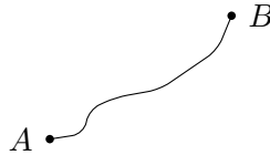
Рис. 15. Траектория муравья
