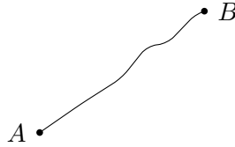
Рис. 15. Траектория муравья
