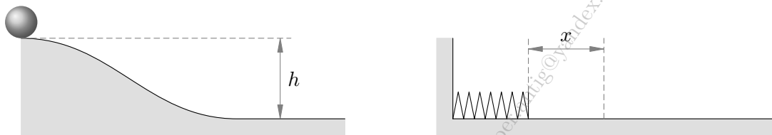
Рис. 55. Шар на горке и сжатая пружина
