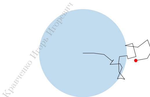
Рис. 65. Броуновское движение
