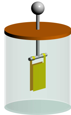
Рис. 92. Электроскоп
