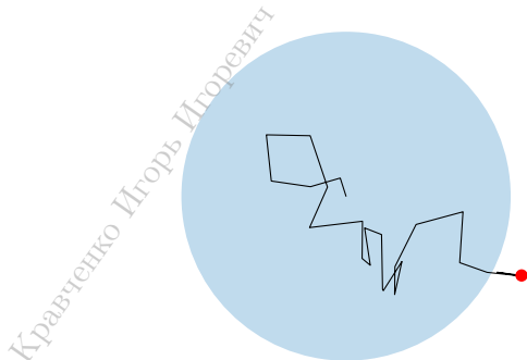
Рис. 67. Броуновское движение
