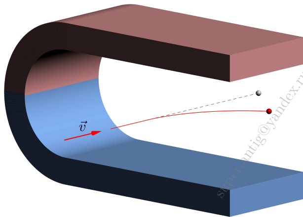
Рис. 153. Отклонение движения заряда в магнитном поле
