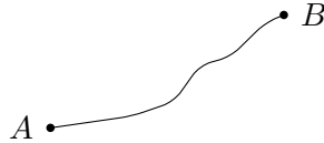
Рис. 15. Траектория муравья
