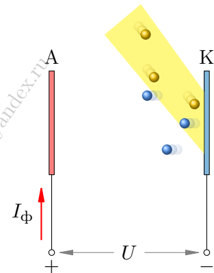
Рис. 195. Фотоэффект
