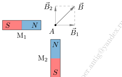
Рис. 140. Принцип суперпозиции магнитных полей
