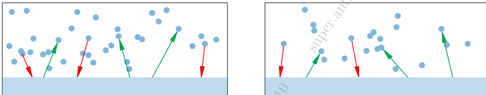
Рис. 72. Пары над жидкостью в сосудах
