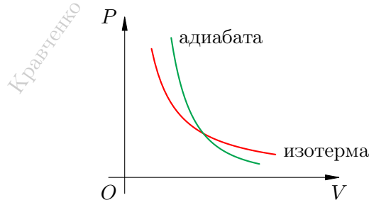
Рис. 84. Адиабата убывает быстрее изотермы
