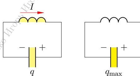
Рис. 162. Электромагнитные колебания в колебательном контуре
