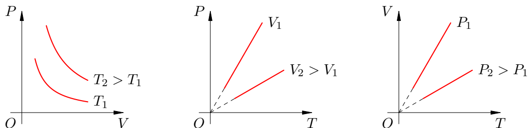
Рис. 69. Графики изопроцессов
