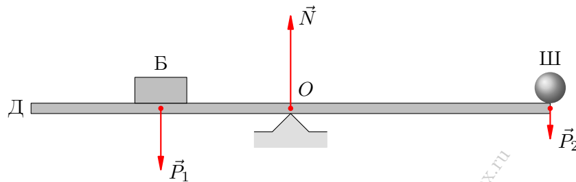
Рис. 43. Равновесие доски
