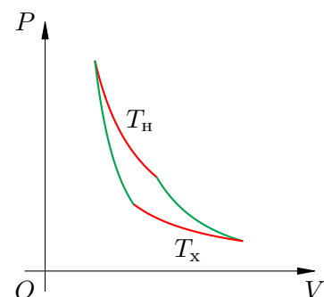
Рис. 86. Цикл Карно
