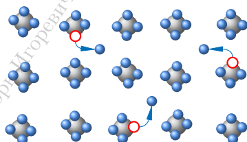
Рис. 127. Появление свободных электронов (и дырок)
