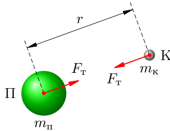
Рис. 34. Притяжение планеты и космического корабля
