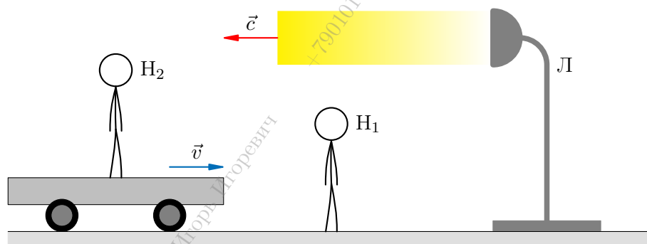
Рис. 204. Наблюдатели фиксируют одинаковую скорость света
