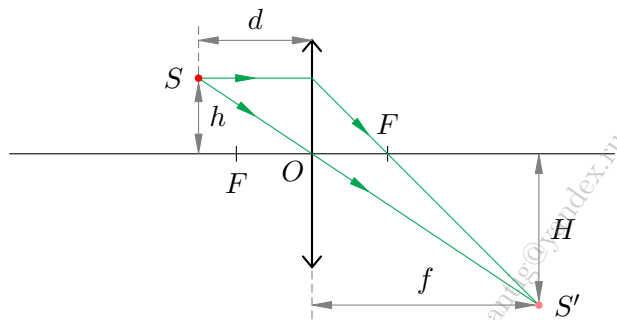
Рис. 184. Построение изображения точки
