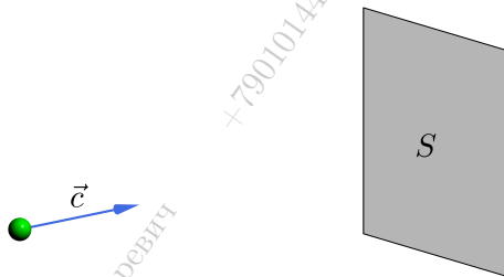
Рис. 197. Падение фотона на поверхность тела
