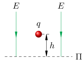
Рис. 100. Заряд в однородном поле
