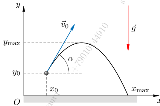
Рис. 19. Полет тела
