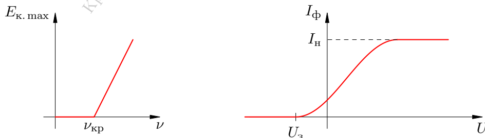
Рис. 195. Зависимости E_{\text{к. max}}(\nu) и I_{\text{ф}}(U) для фотоэффекта
