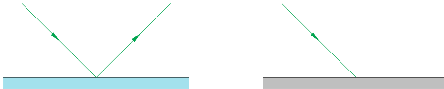
Рис. 196. Падение света на зеркальную и черную поверхность
