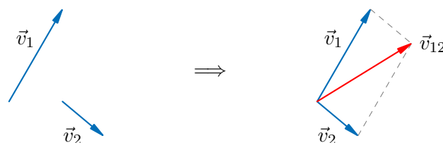
Рис. 3. Правило параллелограмма
