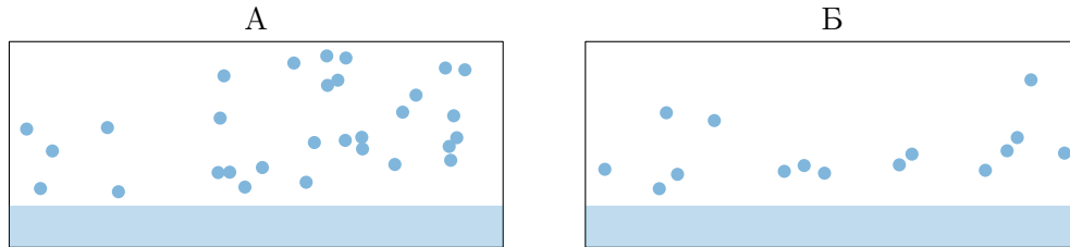
Рис. 73. Пары воды в сосудах
