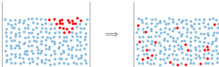
Рис. 66. Диффузия в жидкости
