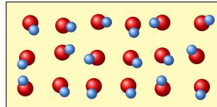
Рис. 110. Диэлектрик
