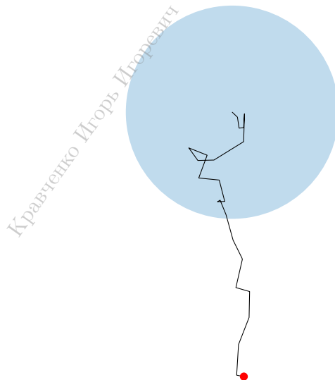
Рис. 65. Броуновское движение
