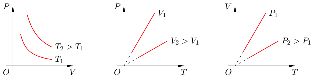
Рис. 69. Графики изопроцессов
