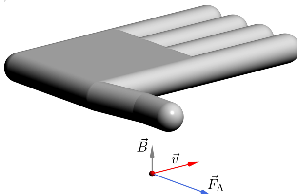
Рис. 152. Правило левой руки
