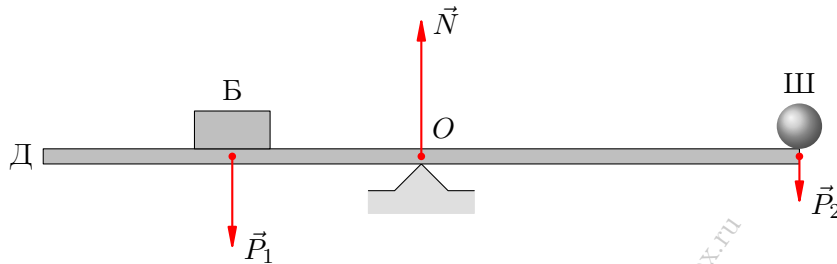
Рис. 43. Равновесие доски
