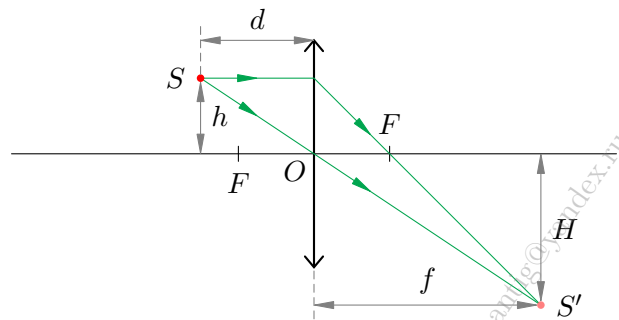
Рис. 182. Построение изображения точки
