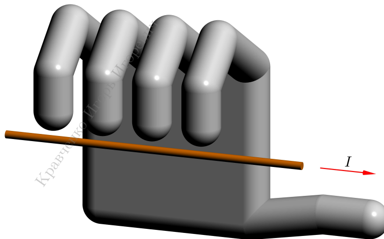
Рис. 144. Правило правой руки
