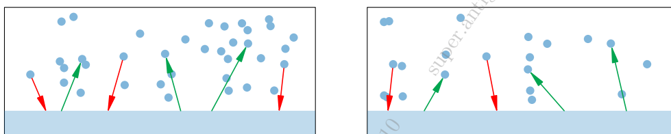
Рис. 70. Пары над жидкостью в сосудах
