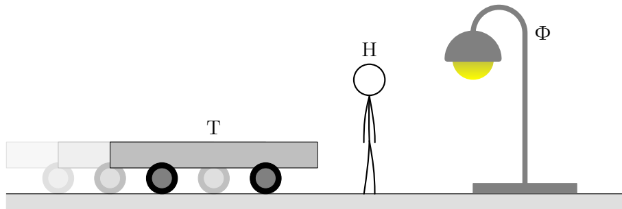
Рис. 4. К определению механического движения
