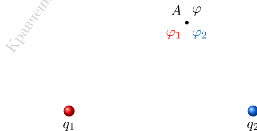
Рис. 103. Принцип суперпозиции для потенциалов
