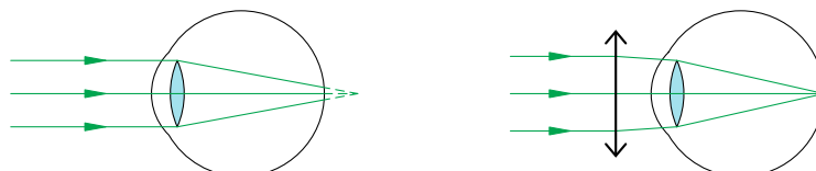
Рис. 185. Дальнозоркость и ее коррекция
