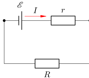
Рис. 123. Полная цепь
