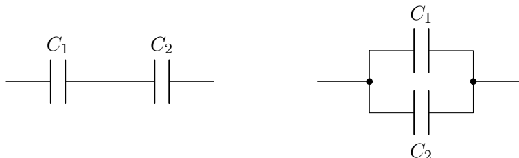
Рис. 113. Последовательное и параллельное соединение двух конденсаторов
