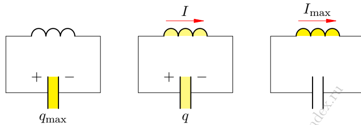
Рис. 161. Электромагнитные колебания в колебательном контуре
