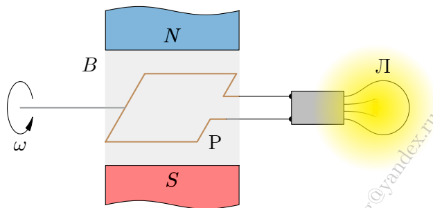
Рис. 166. Схема генератора переменного тока
