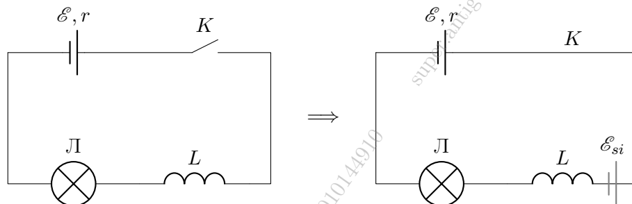
Рис. 160. К опыту по обнаружению явления самоиндукции
