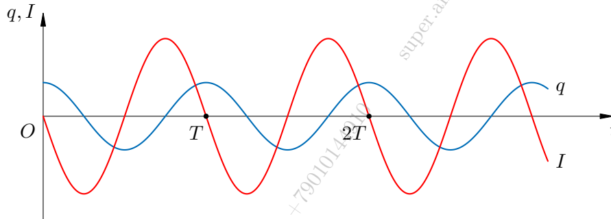
Рис. 163. Графики колебаний заряда и тока в контуре
