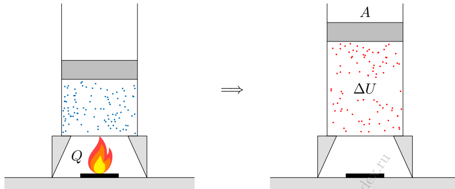
Рис. 81. Газ «на огне»
