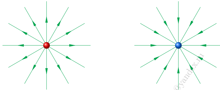
Рис. 96. Линии электрического поля точечного заряда
