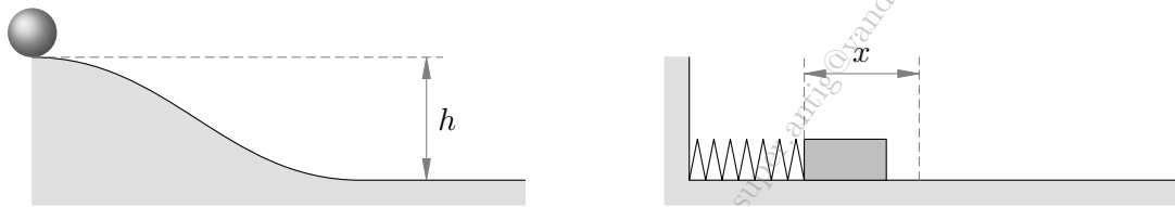
Рис. 56. Начальные положения шара и сжатой пружины с бруском
