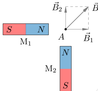
Рис. 138. Принцип суперпозиции магнитных полей
