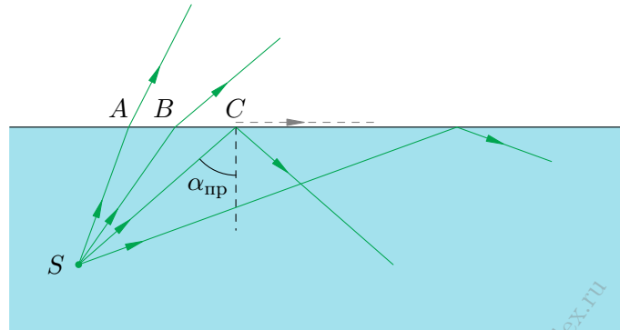
Рис. 175. Полное внутреннее отражение
