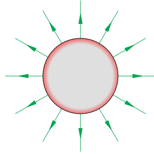
Рис. 108. Линии поля положительно заряженного шара
