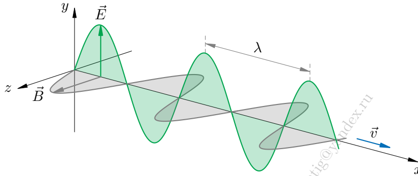
Рис. 168. Электромагнитная волна
