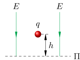
Рис. 98. Заряд в однородном поле
