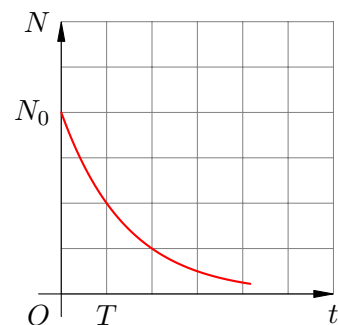
Рис. 202. Зависимость N(t)
