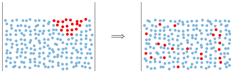
Рис. 64. Диффузия в жидкости
