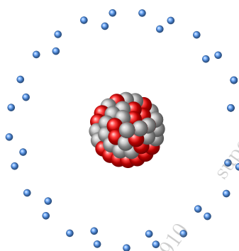
Рис. 85. Модель атома
