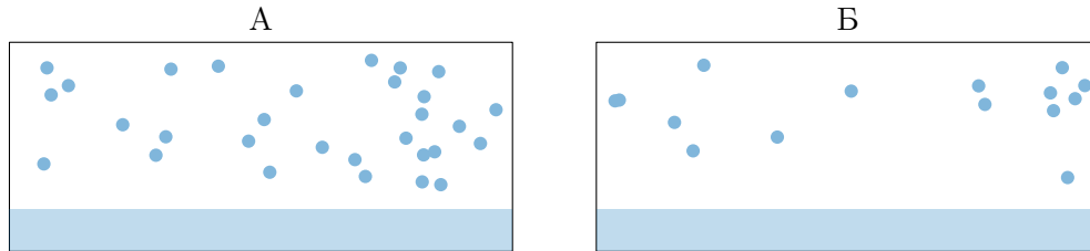
Рис. 71. Пары воды в сосудах
