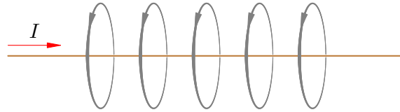
Рис. 143. Линии магнитного поля прямого провода с током
