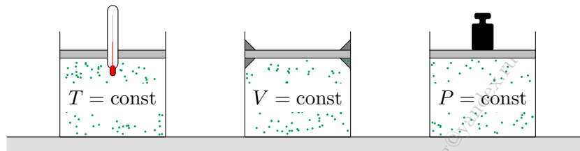
Рис. 68. Газы с разными фиксированными параметрами
