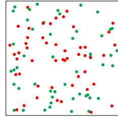
Рис. 66. Два газа в сосуде
