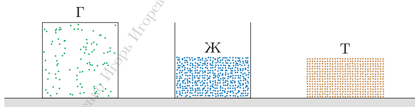
Рис. 63. Модели трех тел
