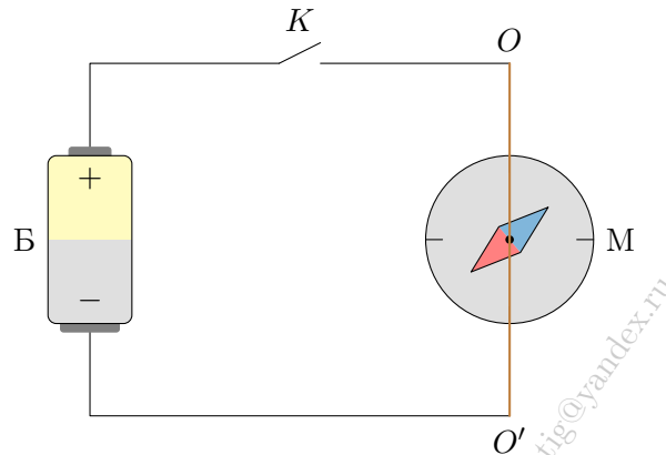
Рис. 141. Опыт Эрстеда: тока в цепи нет
