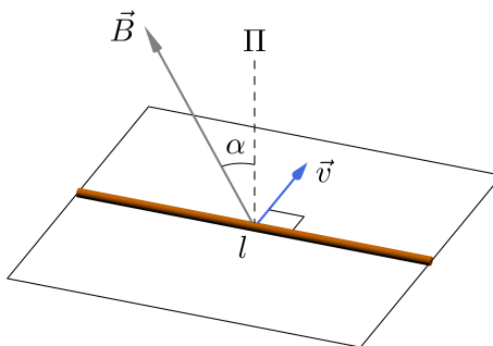
Рис. 158. К определению ЭДС индукции в движущемся проводе
