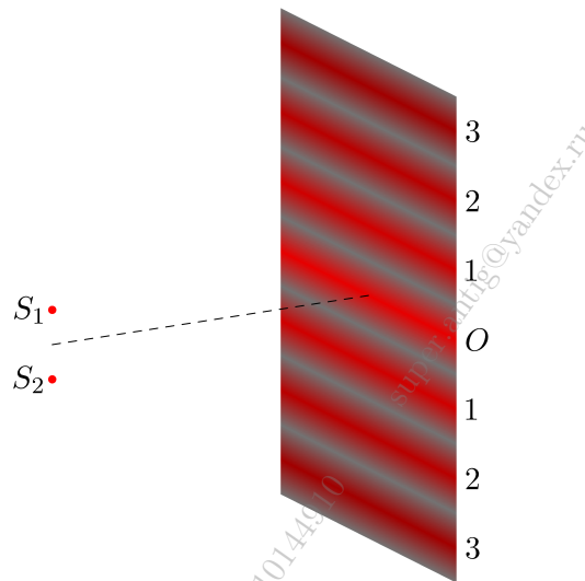
Рис. 187. Интерференция волн двух точечных источников
