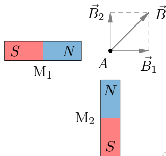
Рис. 140. Принцип суперпозиции магнитных полей
