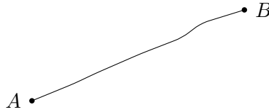
Рис. 15. Траектория муравья
