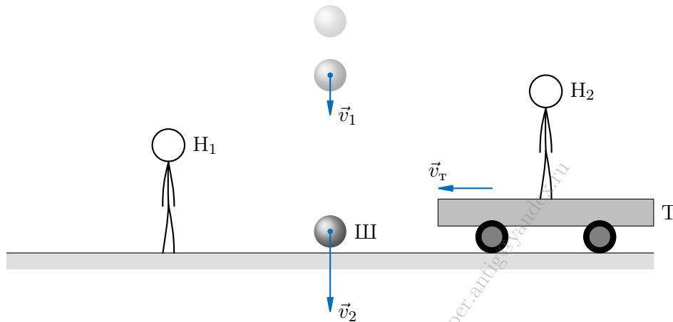
Рис. 25. Наблюдатели и падающий шар
