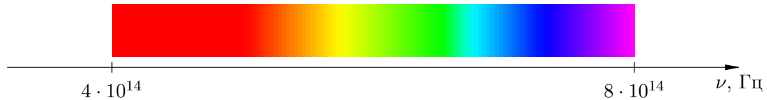
Рис. 192. Спектр белого света
