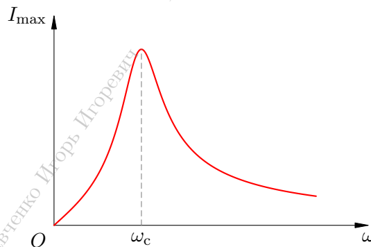
Рис. 167. Резонансная кривая
