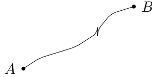
Рис. 15. Траектория муравья
