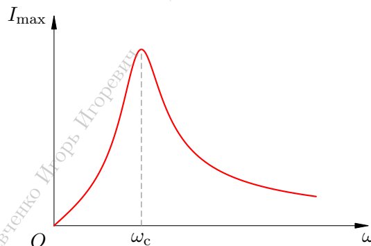
Рис. 165. Резонансная кривая
