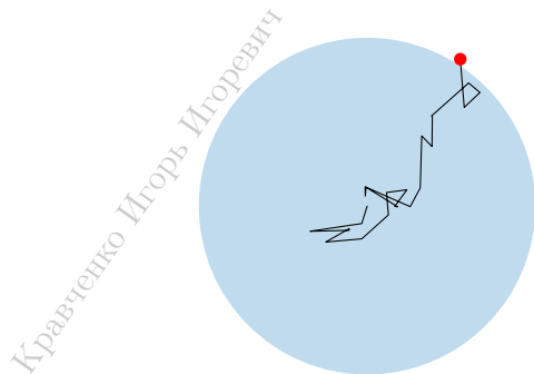
Рис. 65. Броуновское движение
