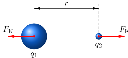
Рис. 95. Взаимодействие двух отрицательных зарядов
