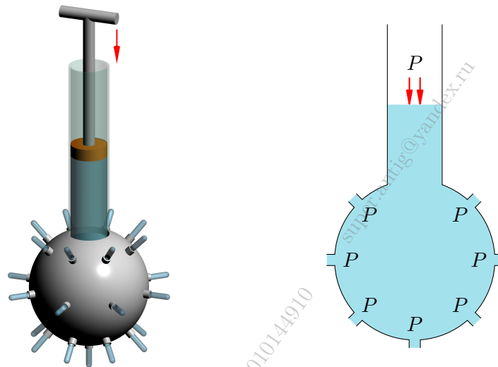
Рис. 45. Шар Паскаля
