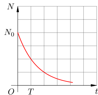
Рис. 202. Зависимость N(t)
