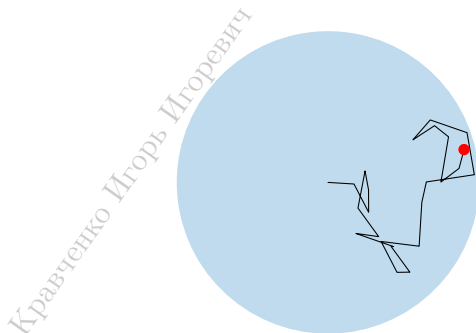
Рис. 65. Броуновское движение
