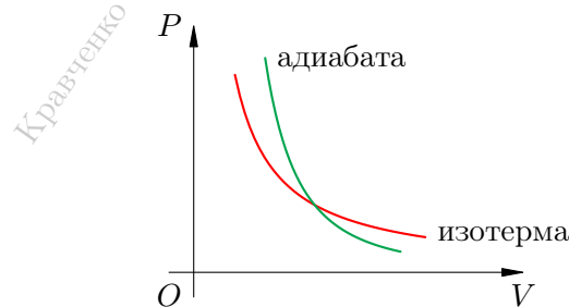
Рис. 82. Адиабата убывает быстрее изотермы
