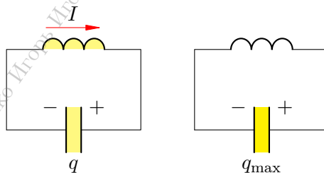
Рис. 164. Электромагнитные колебания в колебательном контуре
