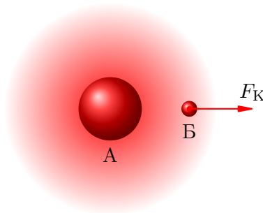
Рис. 96. Действие поля одного заряда на другой
