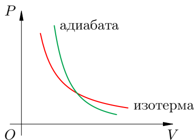
Рис. 82. Адиабата убывает быстрее изотермы
