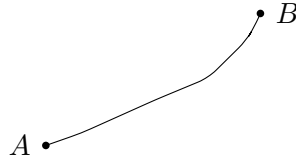
Рис. 15. Траектория муравья
