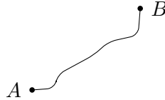
Рис. 15. Траектория муравья
