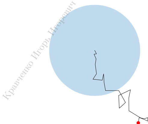
Рис. 65. Броуновское движение
