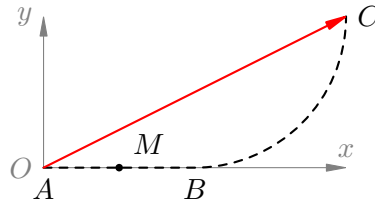
Рис. 6. Движение материальной точки
