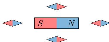
Рис. 135. Установление магнитных стрелок возле магнита
