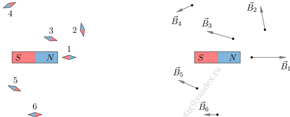
Рис. 136. Стрелки и соответствующие векторы индукции
