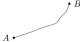
Рис. 15. Траектория муравья
