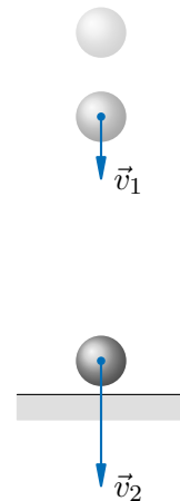
Рис. 18. Падение шара
