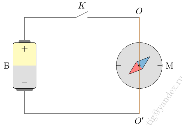
Рис. 141. Опыт Эрстеда: тока в цепи нет
