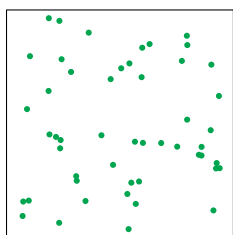
Рис. 67. Газы по отдельности
