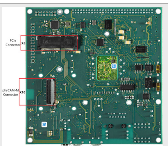
图 2: phyBOARD-Polis 器件 (底部)
