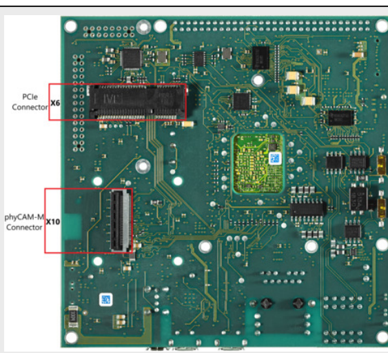
图 2: phyBOARD-Polis 器件 (底部)
