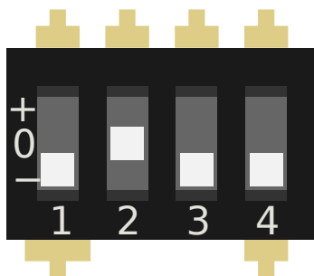
图 6: JTAG mode
