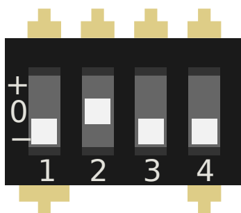
图 6: JTAG mode
