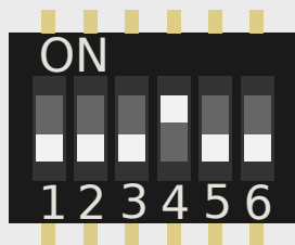
图 8: UART1 RS485
