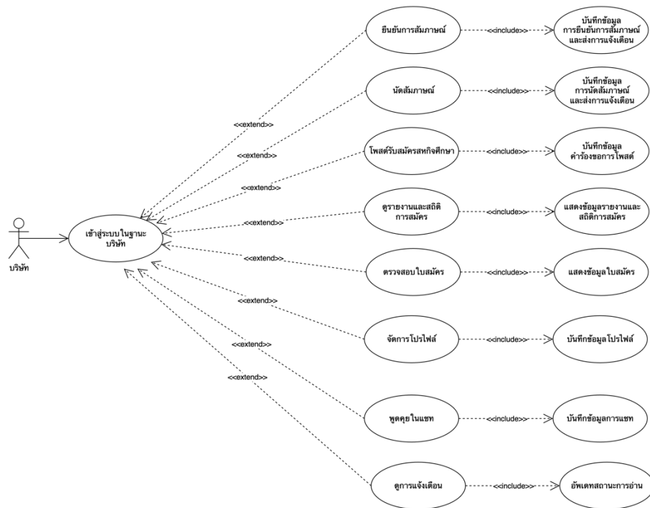
รูปที่ 3.4 System Use Case Diagram - Company
