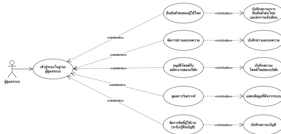
รูปที่ 3.8 System Use Case Diagram - Admin
