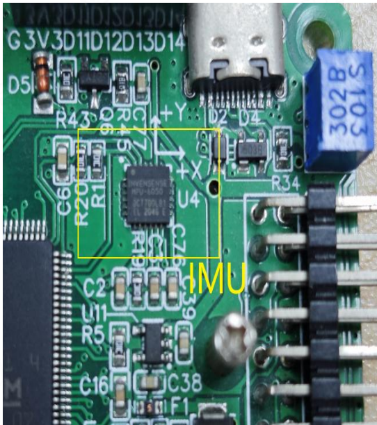
图 1-2 ROS 教育机器人上的 IMU 位置
