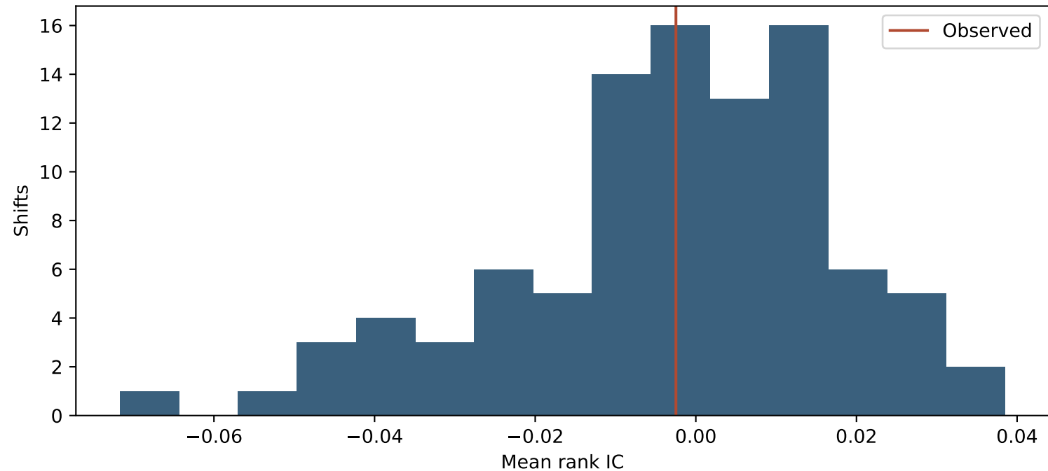
Circular-shift placebo; p=0.558
