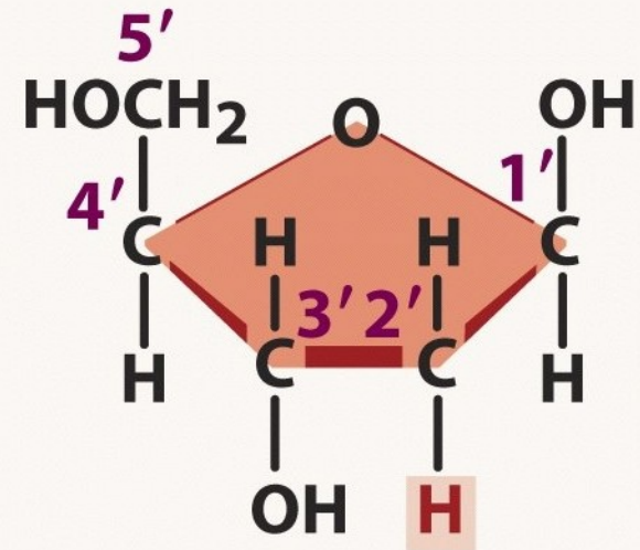
Deoxyribose
