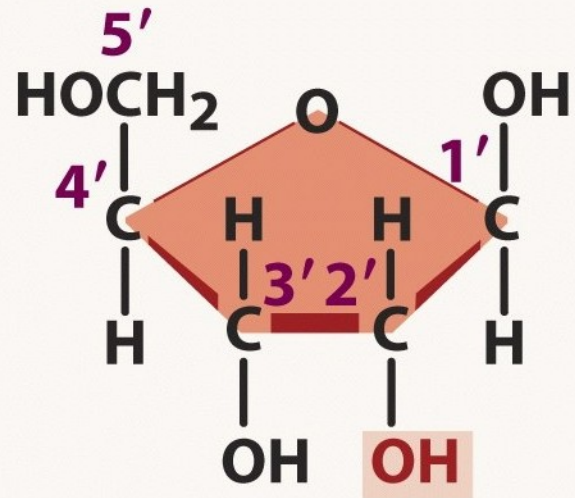
Ribose
