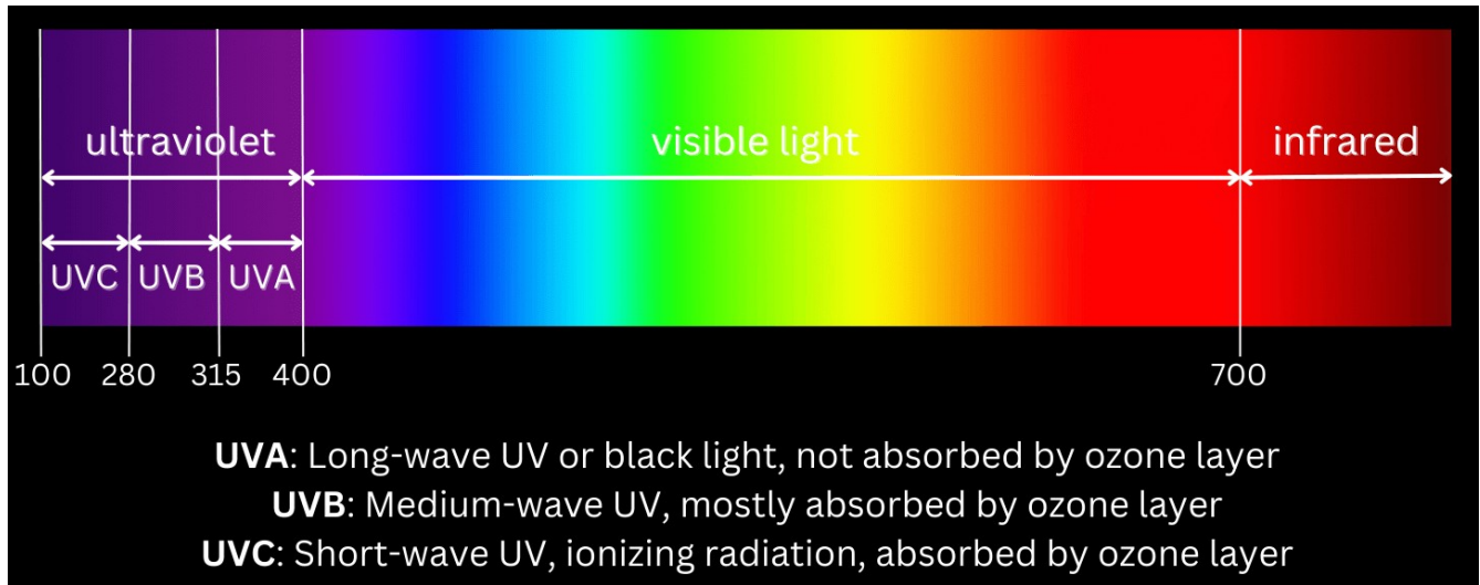
Figura E7.5 La luce ultravioletta è la porzione dello spettro elettromagnetico la cui lunghezza d'onda è minore di quella della luce visibile ma maggiore di quella dei raggi X.
